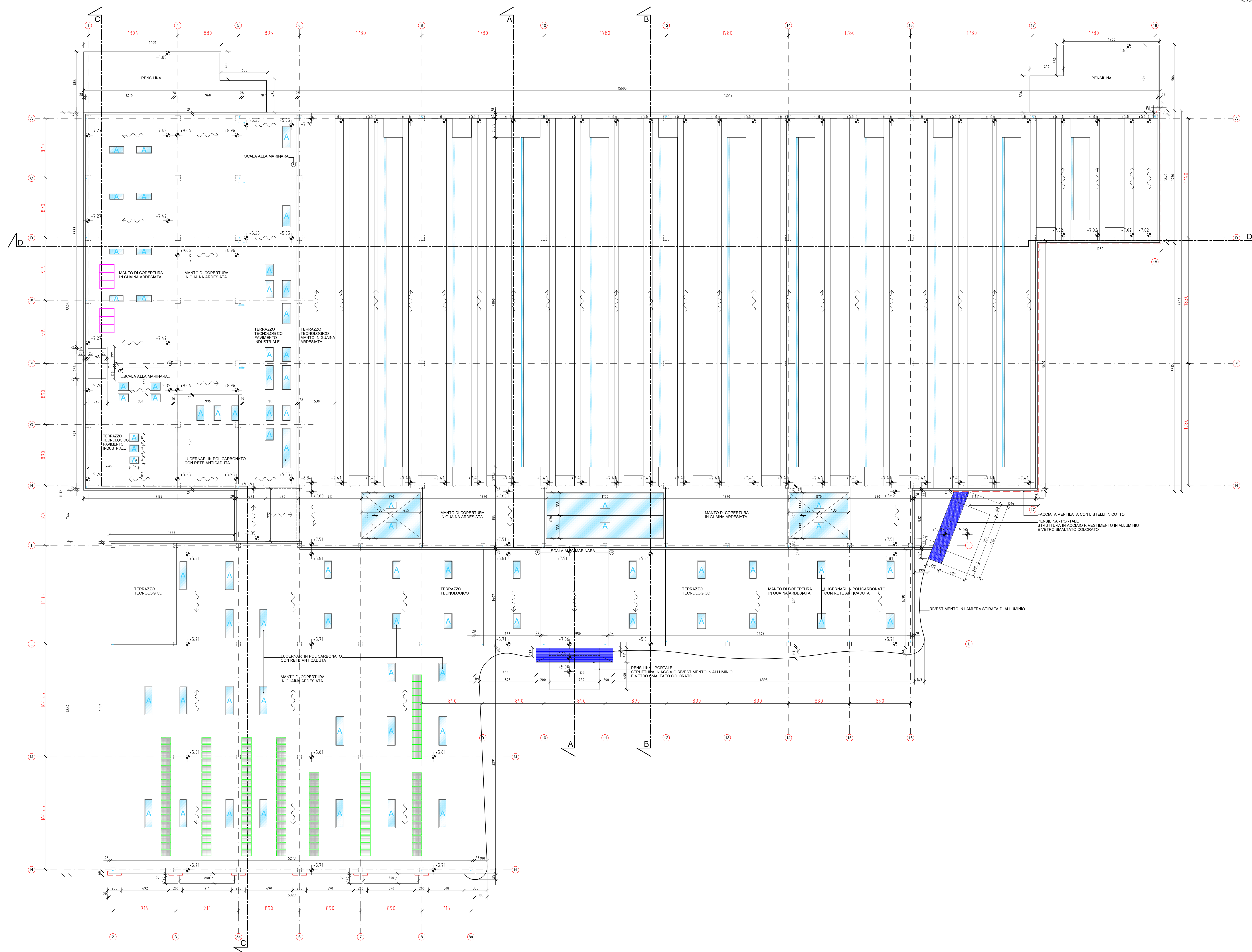
PIANTA COPERTURA SCALA 1:200
