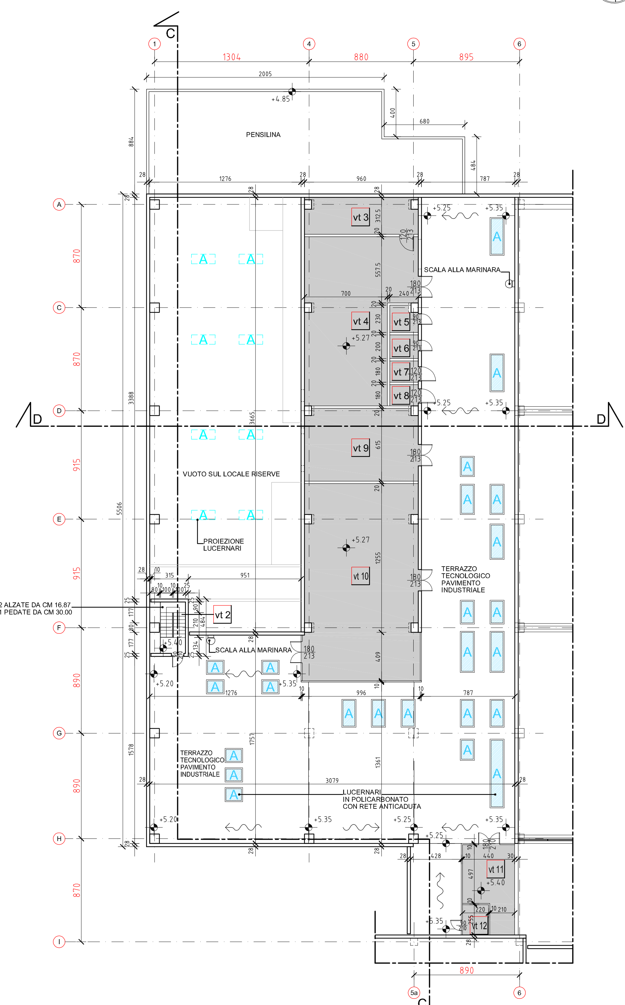
PIANTA PRIMO PIANO SCALA 1:200
