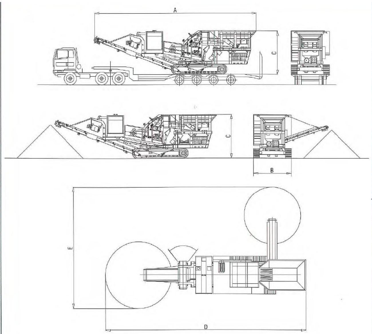
Figura 3: Schede tecniche dei frantoi – Marca: MEM – Mod: BRS/75.50.1
