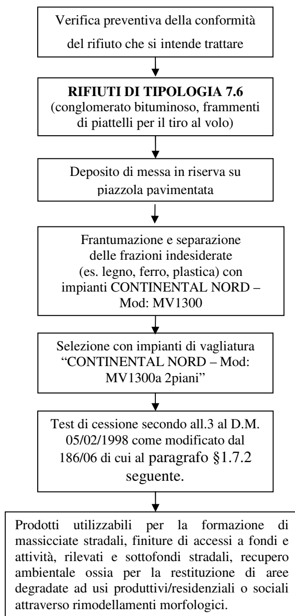
Figura 6: Schema a blocchi delle attività di recupero tipologia 7.6
