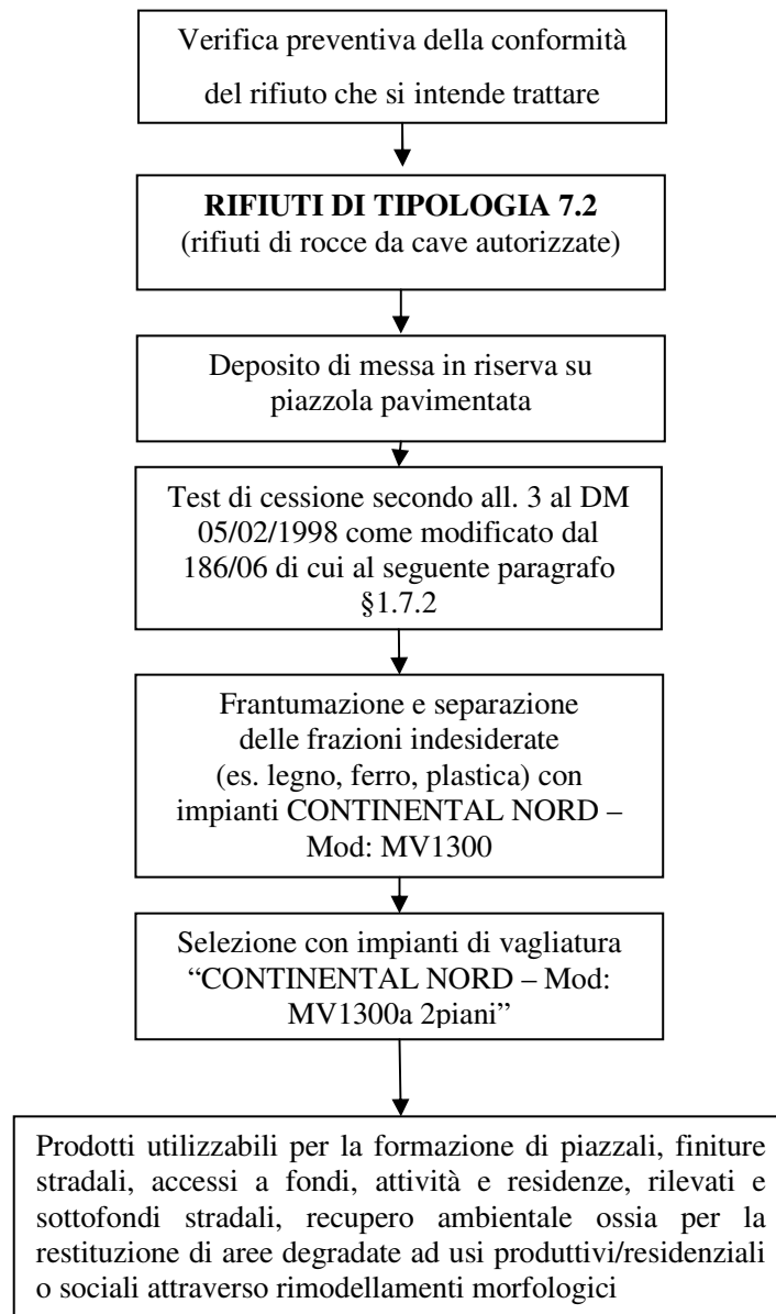
Figura 5: Schema a blocchi delle attività di recupero tipologia 7.2
