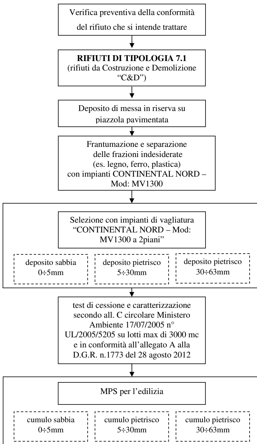
Figura 4: Schema a blocchi delle attività di recupero tipologia 7.1
