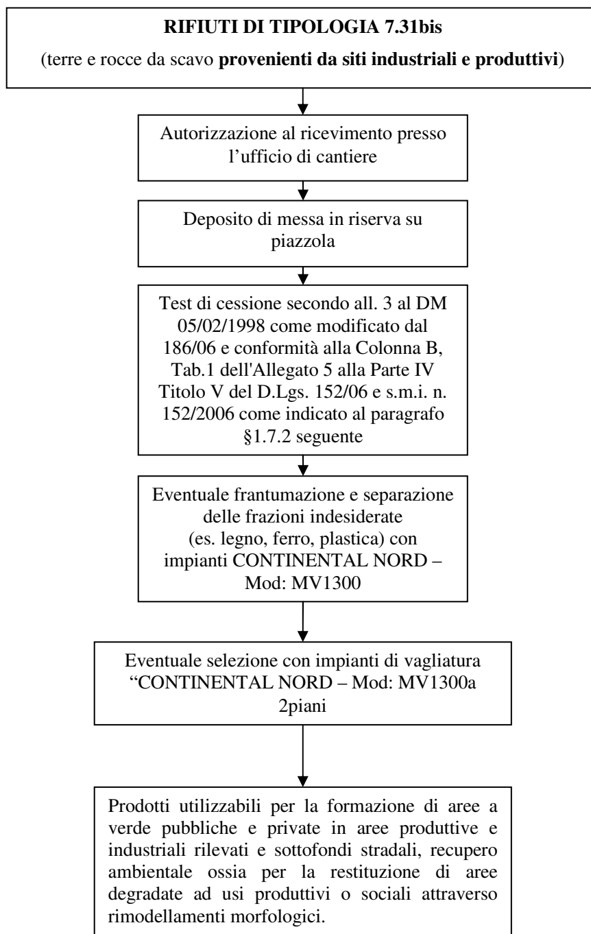
Figura 8: Schema a blocchi delle attività di recupero tipologia 7.31bis (Colonna B)
