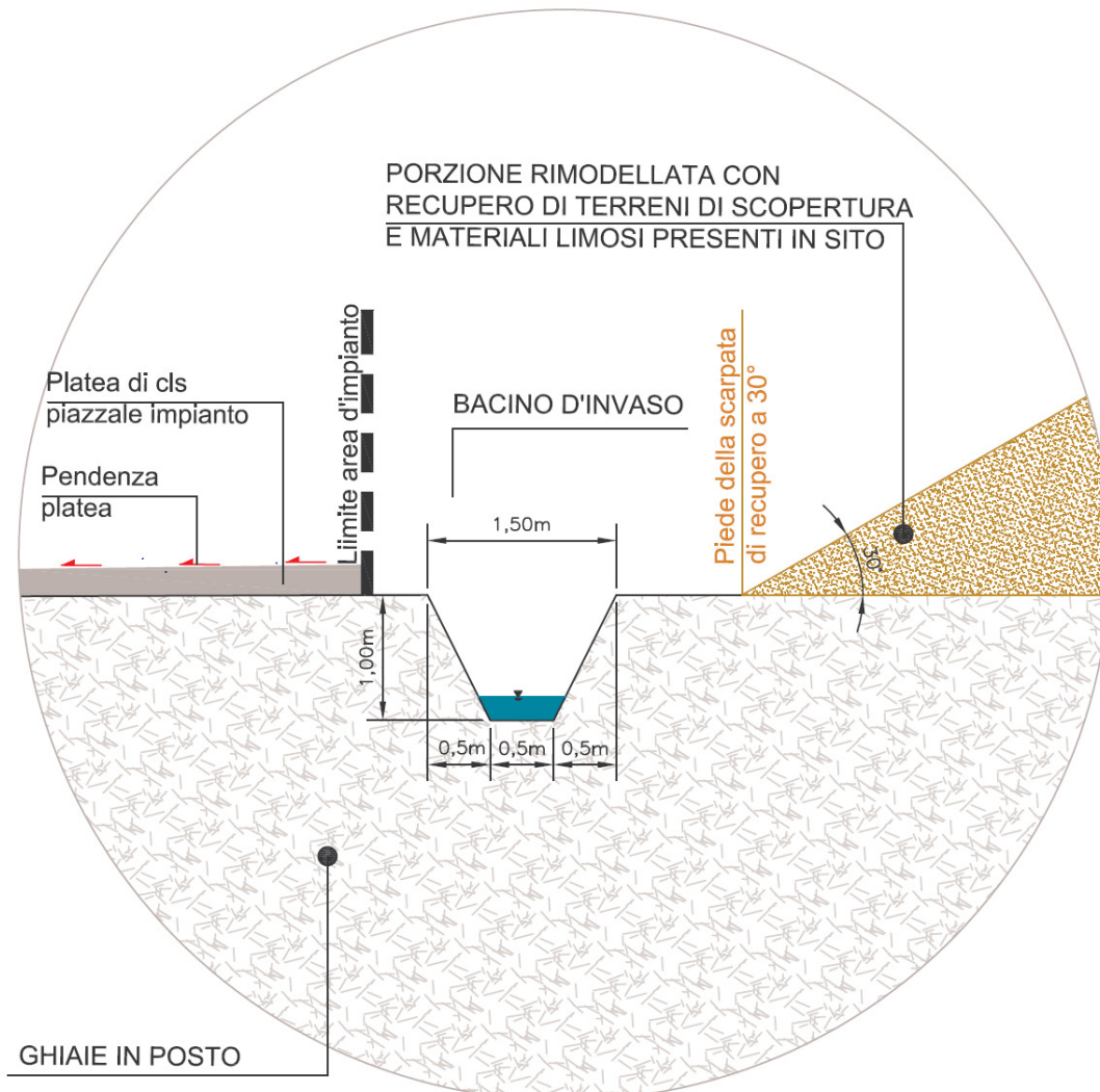
Figura 13: Layout di gestione acque meteoriche, e relativi particolari
