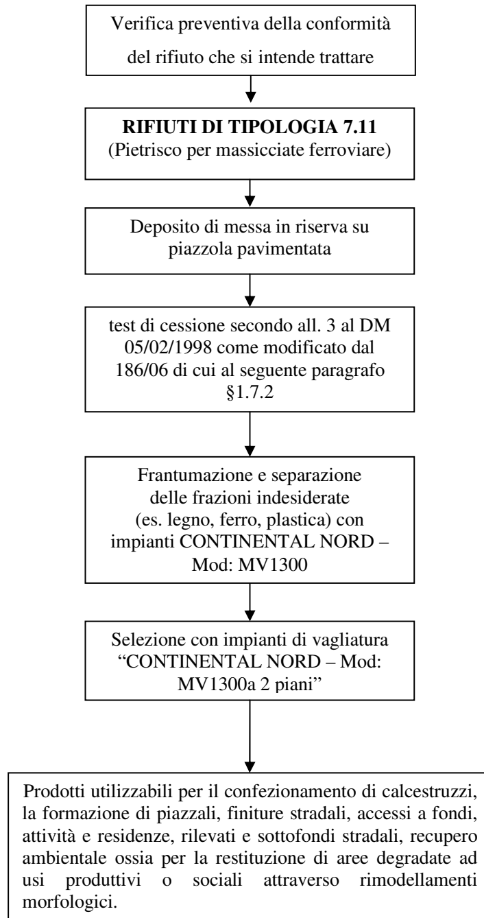
Figura 9: Schema a blocchi delle attività di recupero tipologia 7.11
