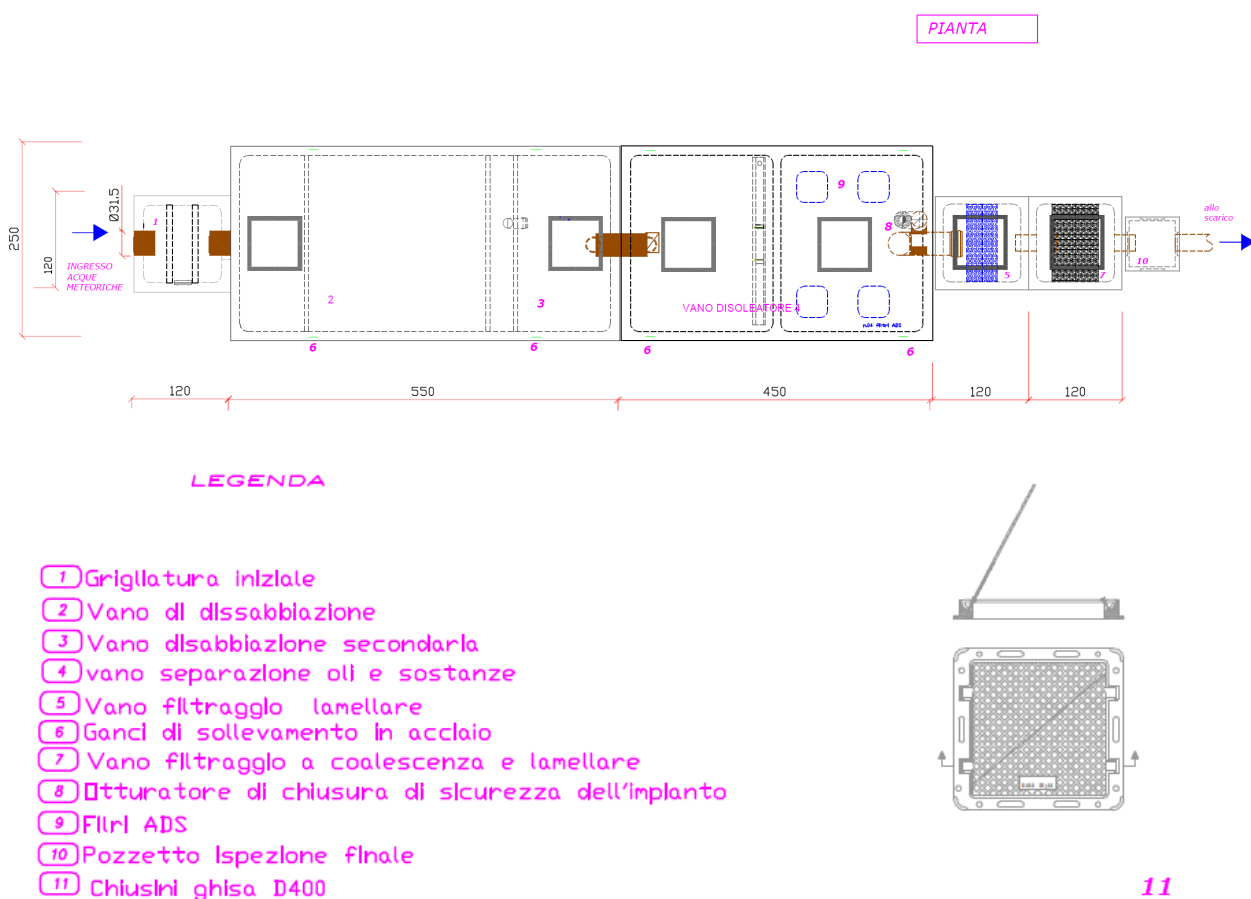
Figura 11: Schede dell'impianto di depurazione.
