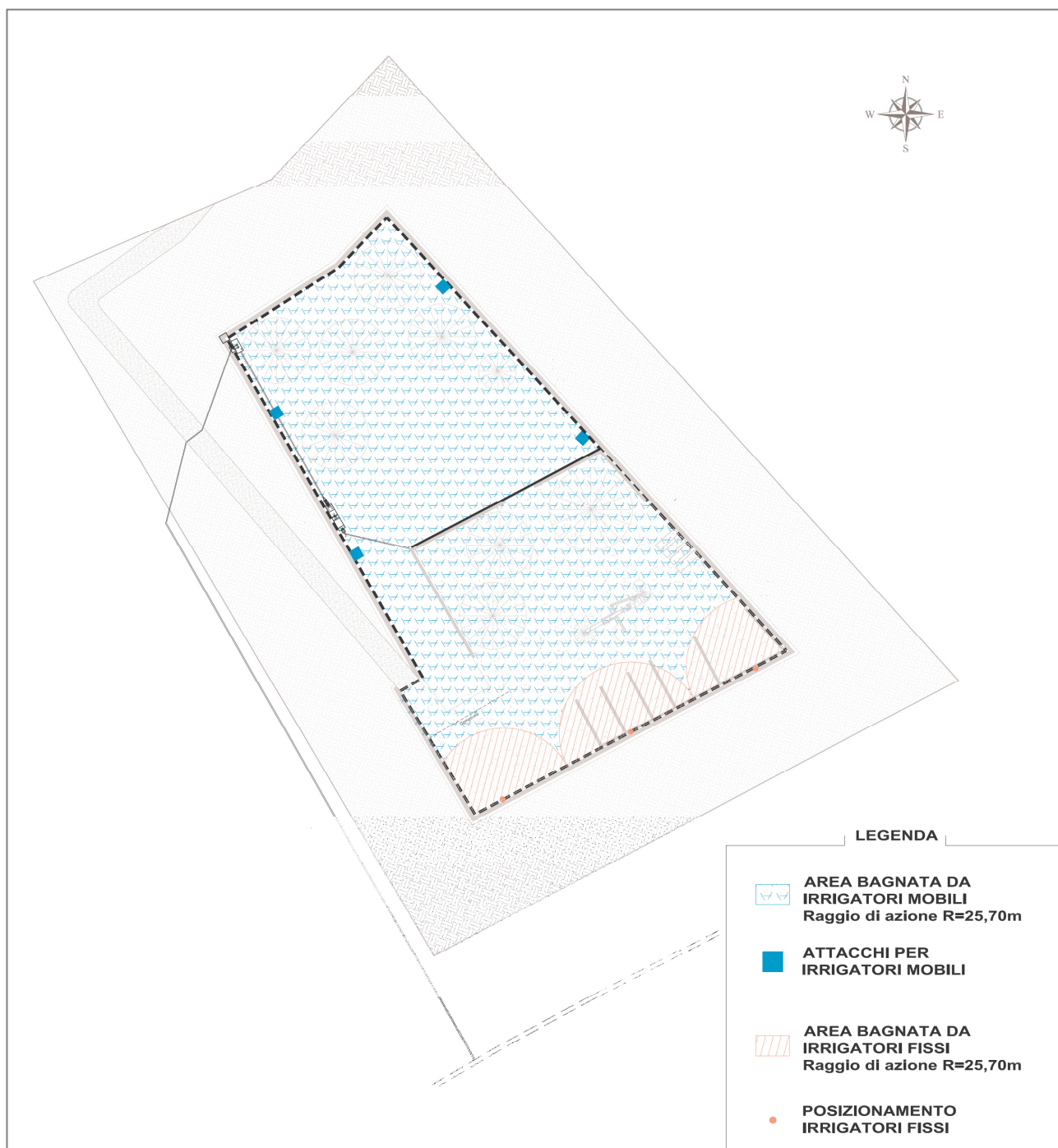
Figura 14: Layout con indicazione impianto di irrigazione per l'abbattimento delle emissioni in atmosfera
