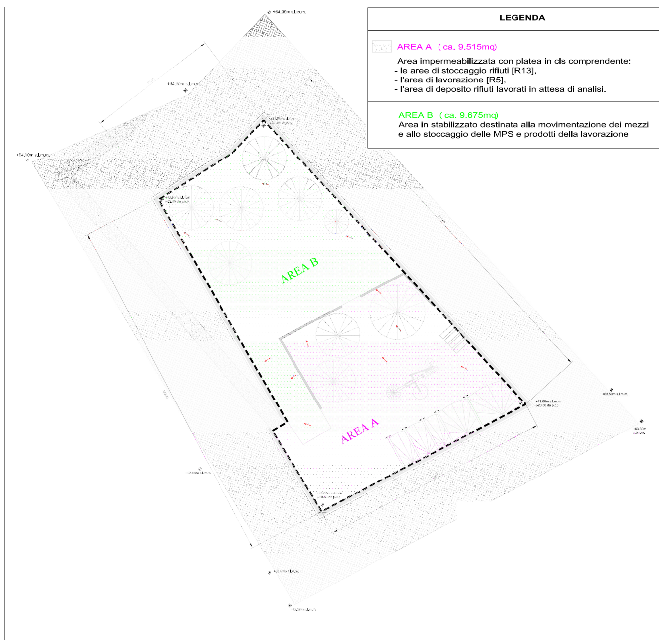
Figura 1: Layout di progetto
