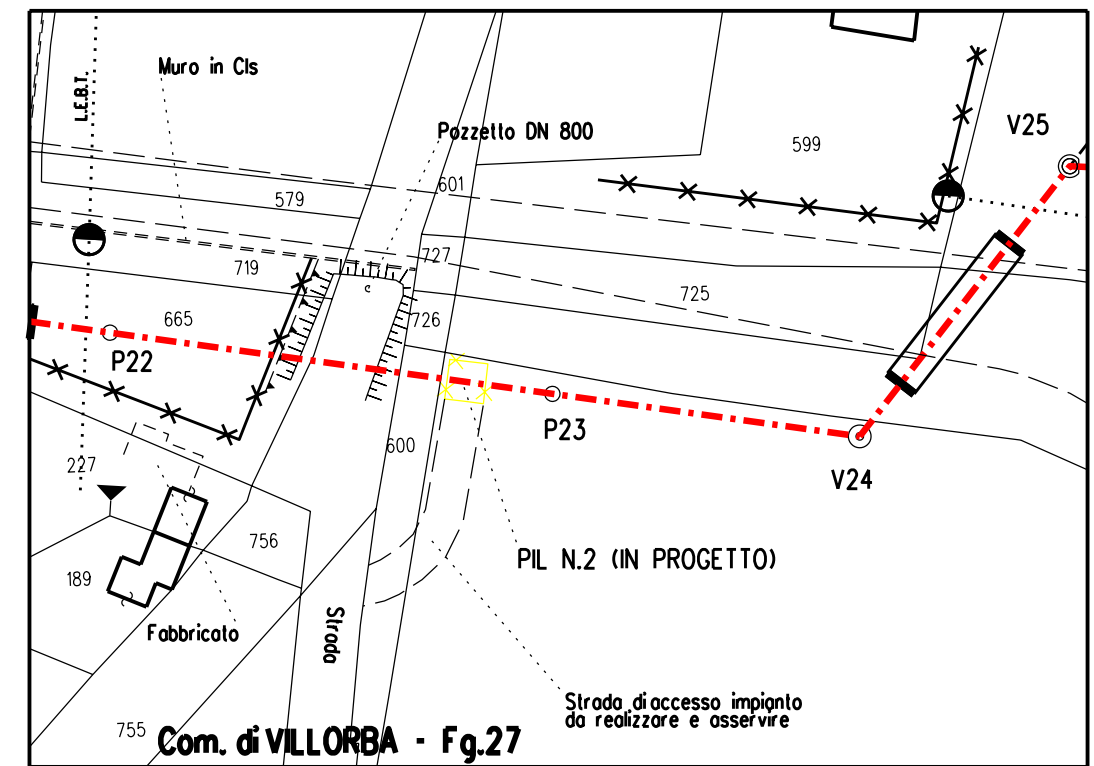
STRALCIO PLANIMETRICO 1:1000
