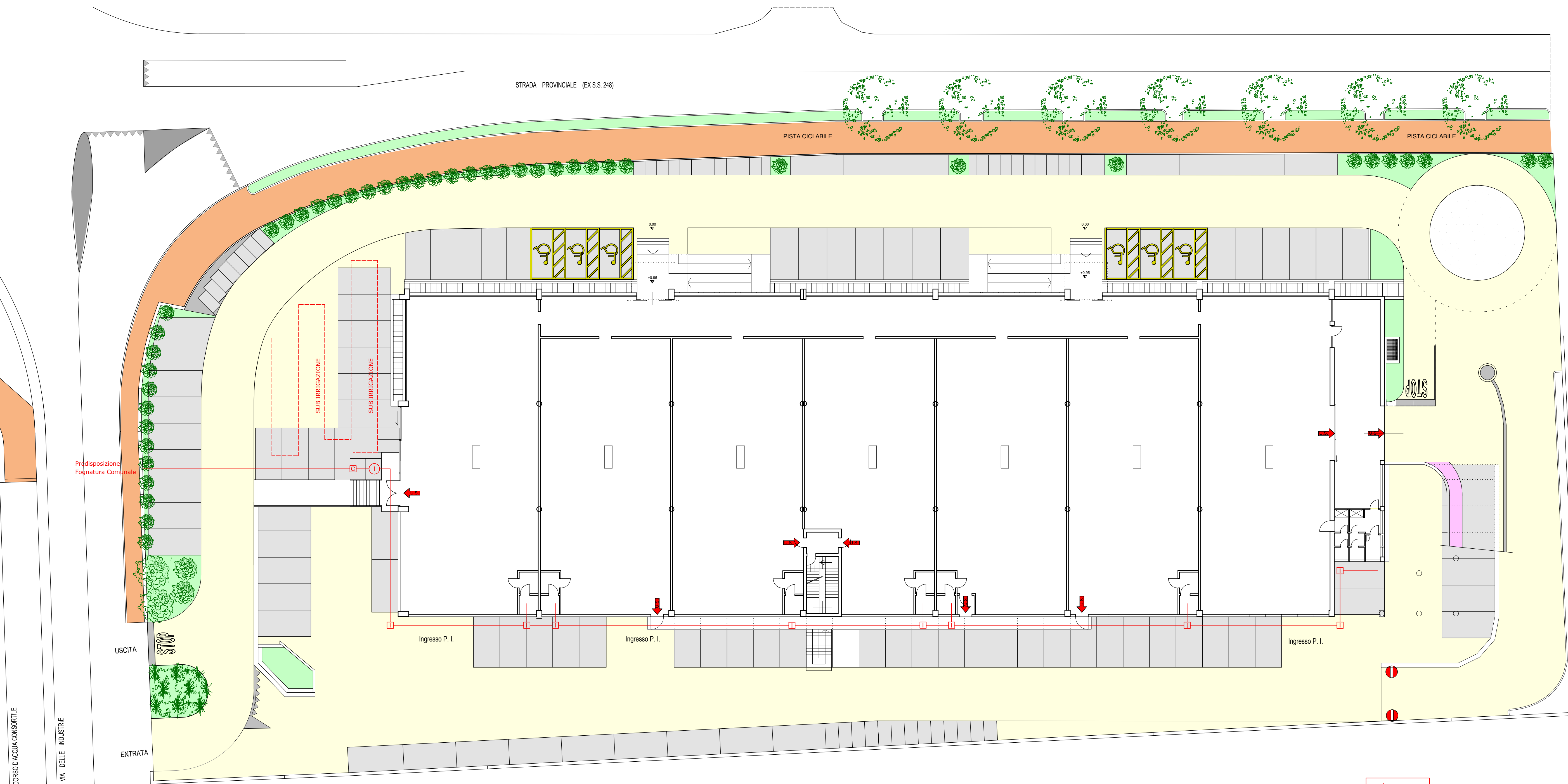
PIANTA PIANO TERRA E SISTEMAZIONI ESTERNE scala 1:200
