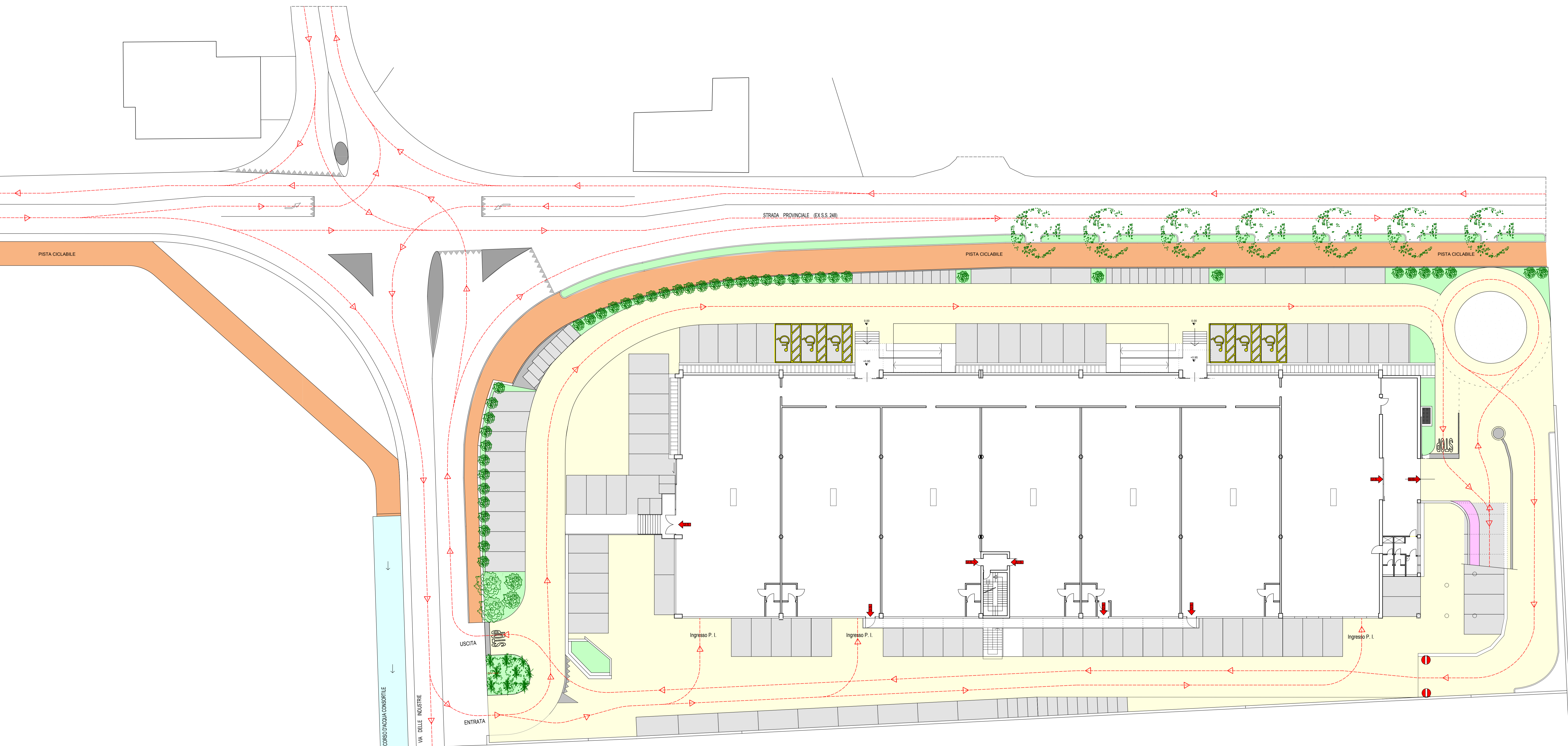
PIANTA PIANO TERRA E SISTEMAZIONI ESTERNE scala 1:200
