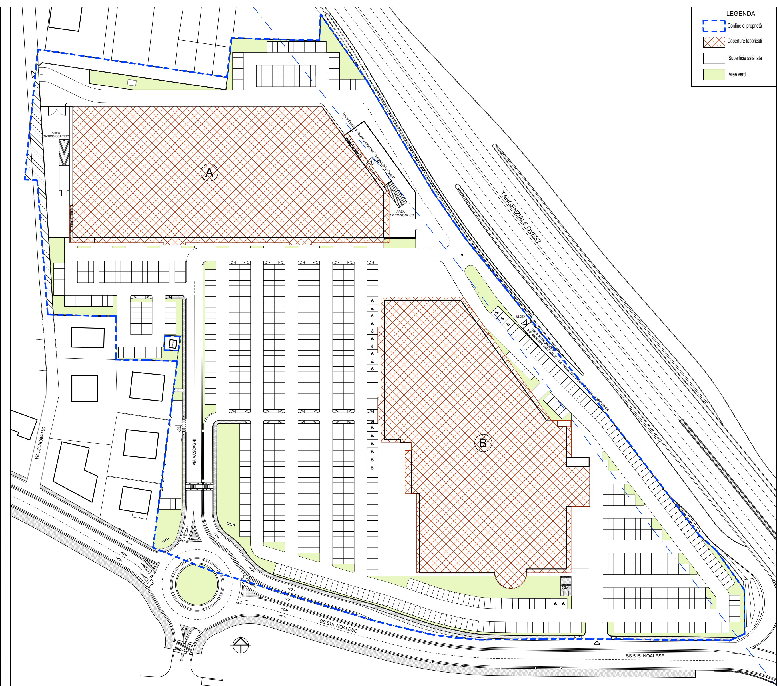
PLANIMETRIA - VARIANTE- DIMOSTRAZIONE SUPERFICIE IMPERMEABILE - scala 1:1000
