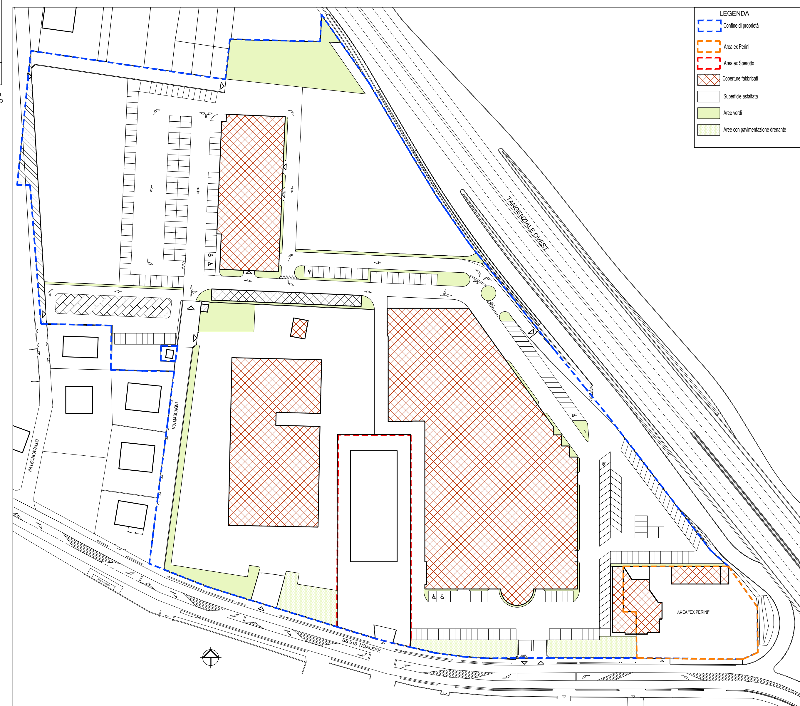
PLANIMETRIA - STATO DI FATTO - DIMOSTRAZIONE SUPERFICIE IMPERMEABILE - scala 1:1000
