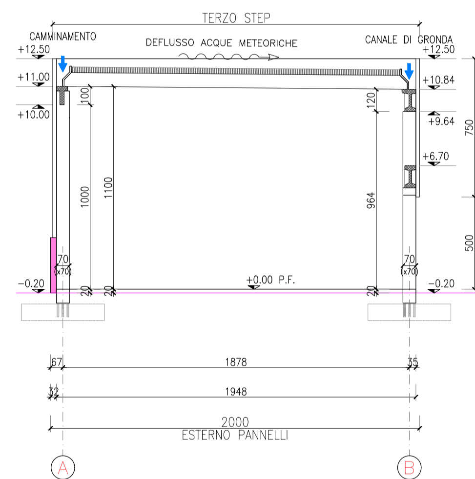
SEZIONE A-A
