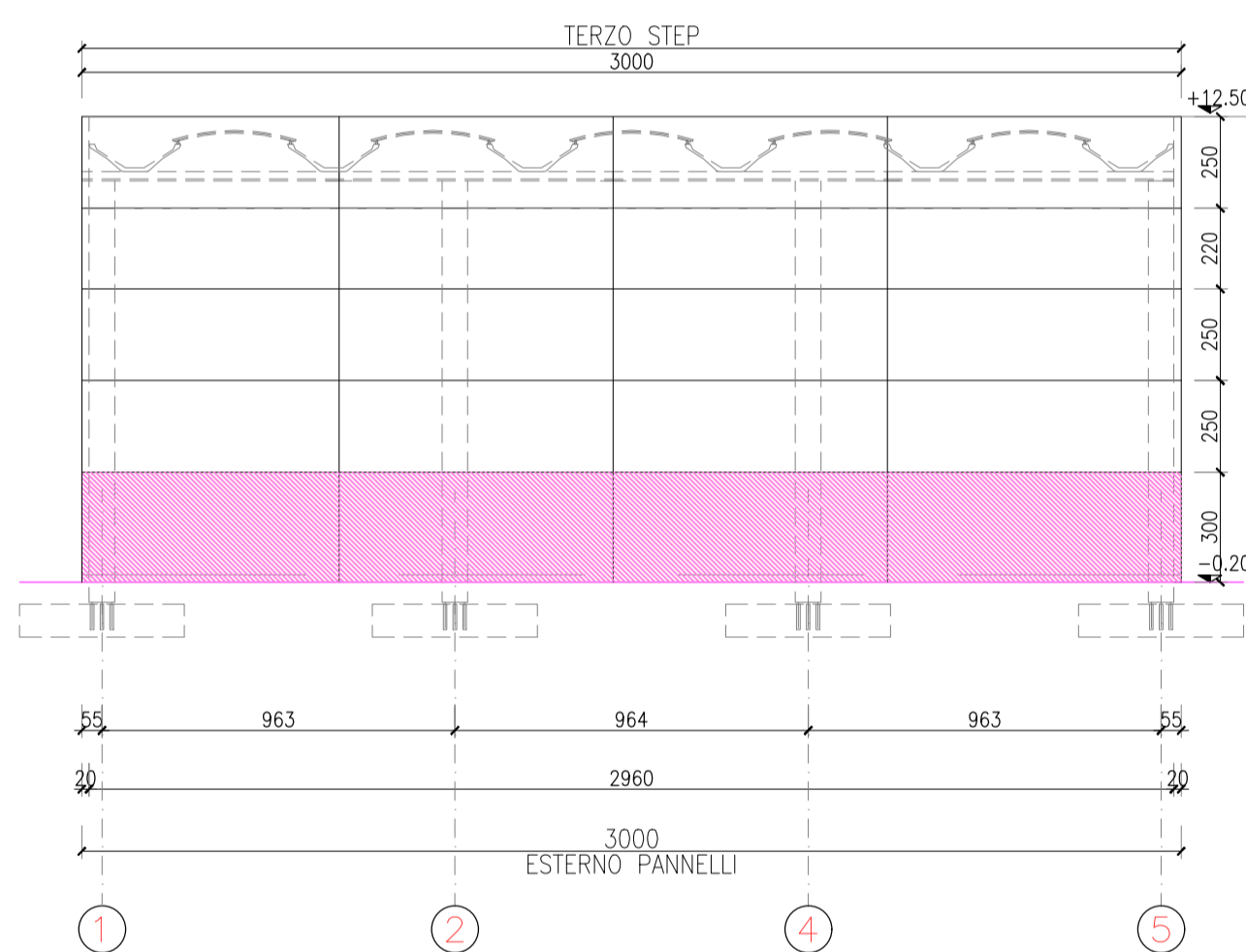
PROSPETTO OVEST
