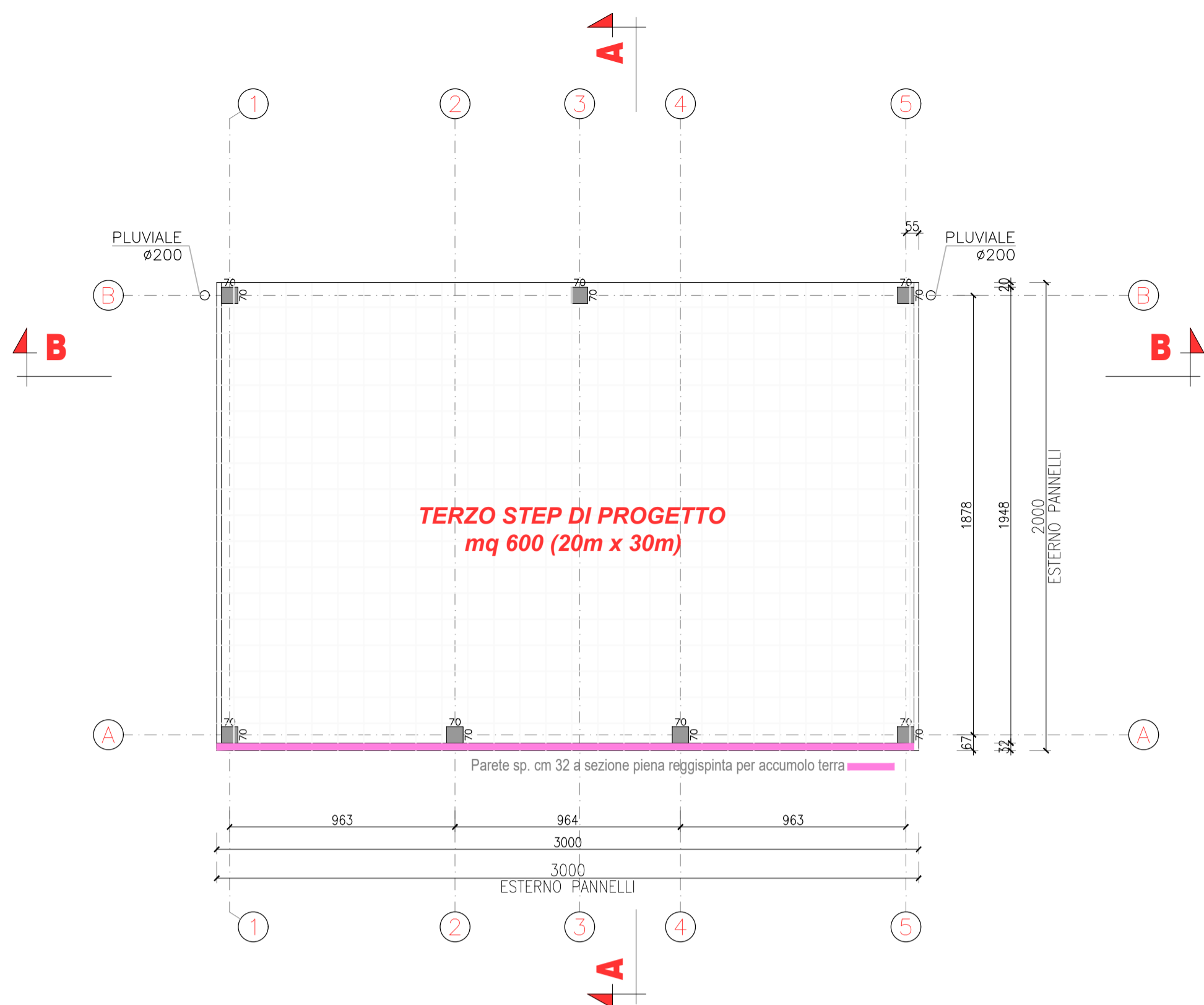
PIANTA PILASTRI
