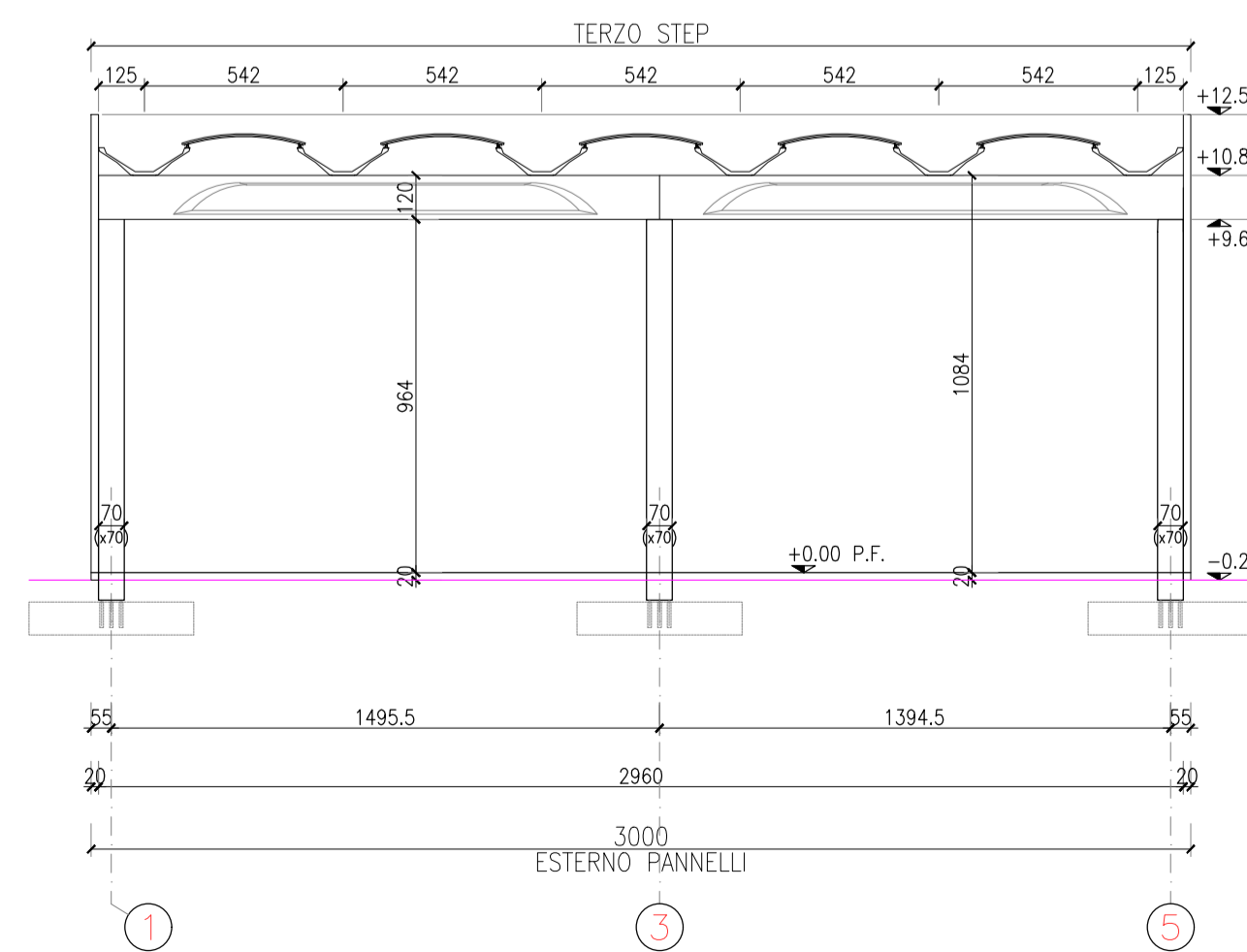
SEZIONE B-B
