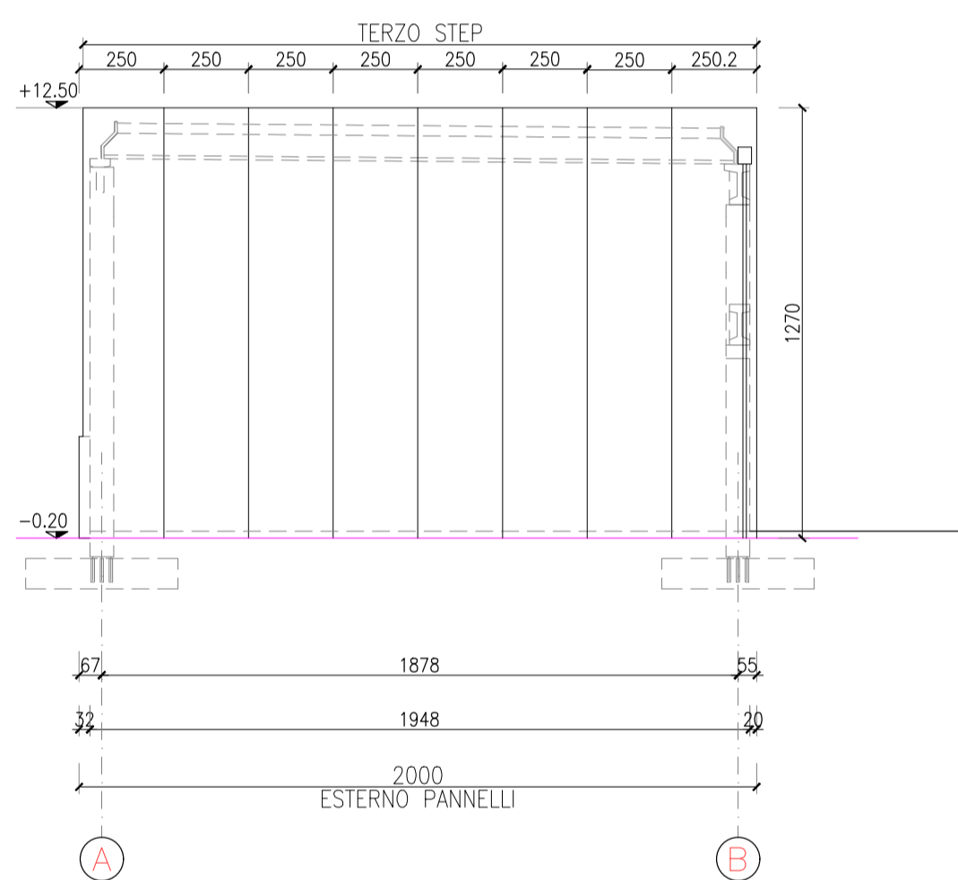
PROSPETTO SUD
