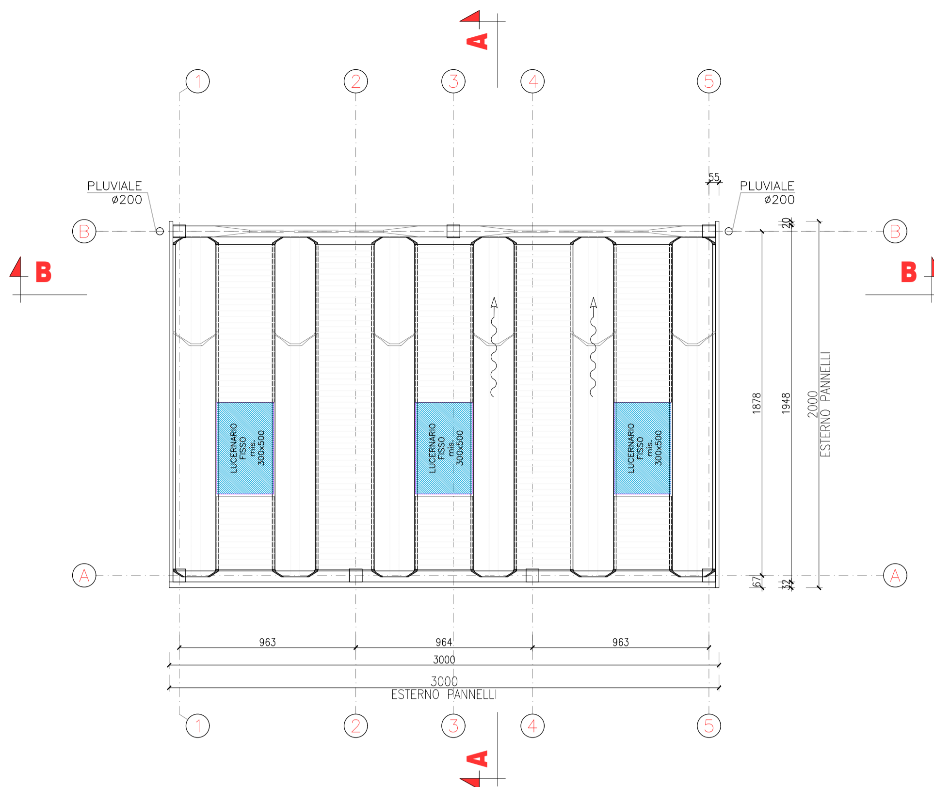
PIANTA COPERTURA
