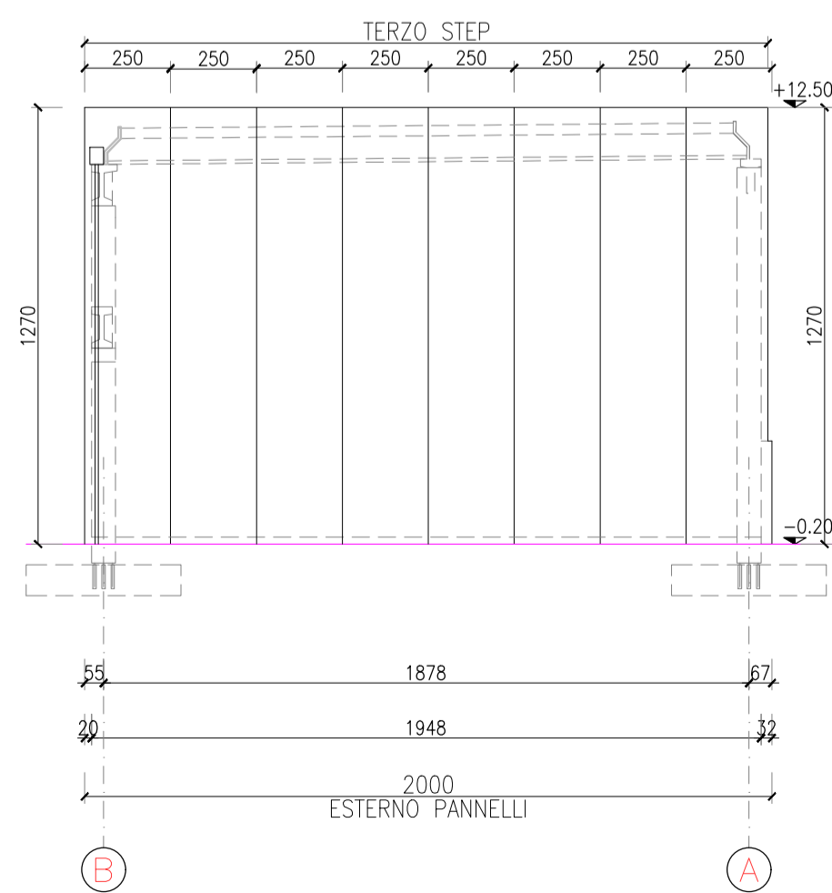
PROSPETTO NORD
