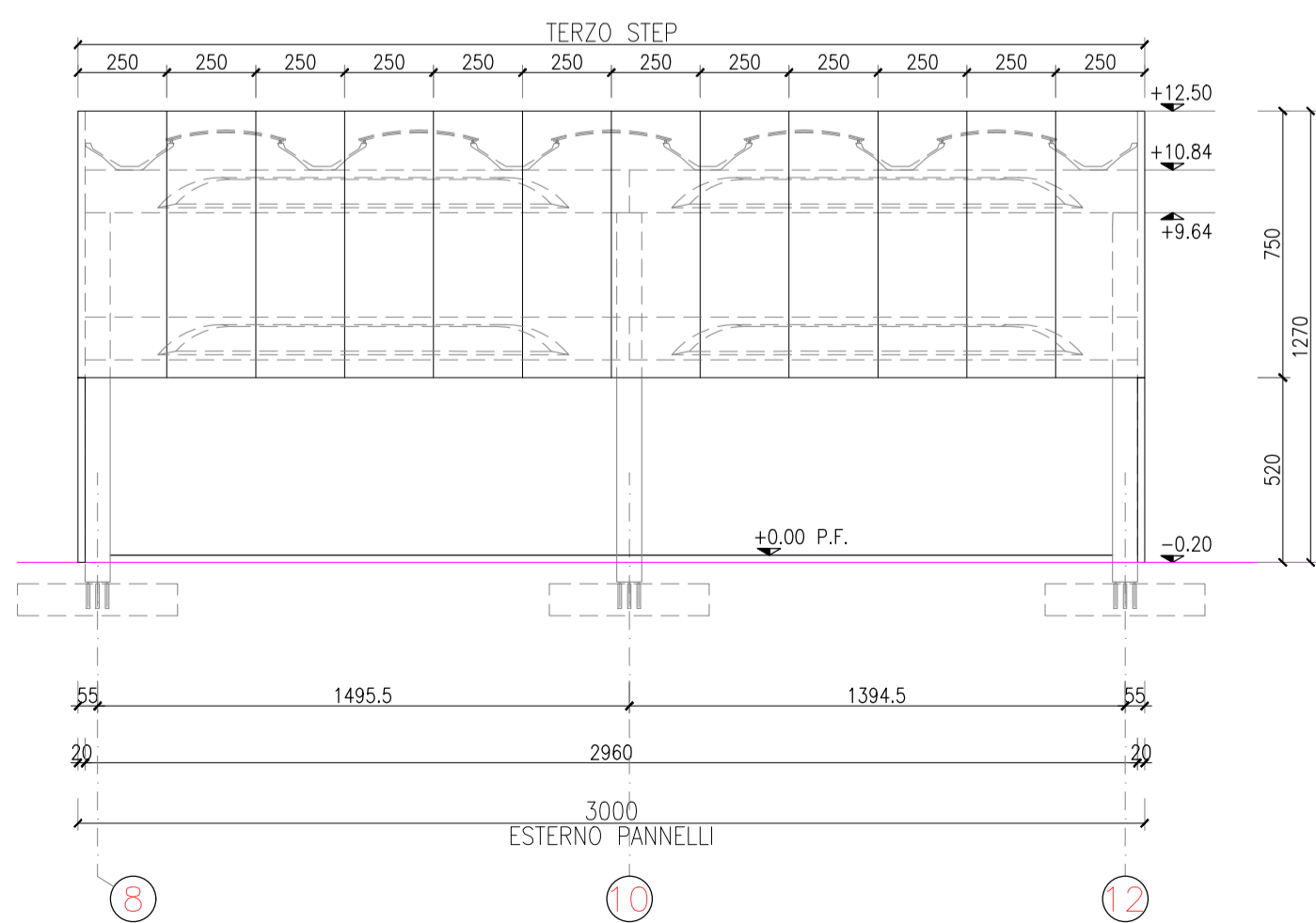
PROSPETTO EST
