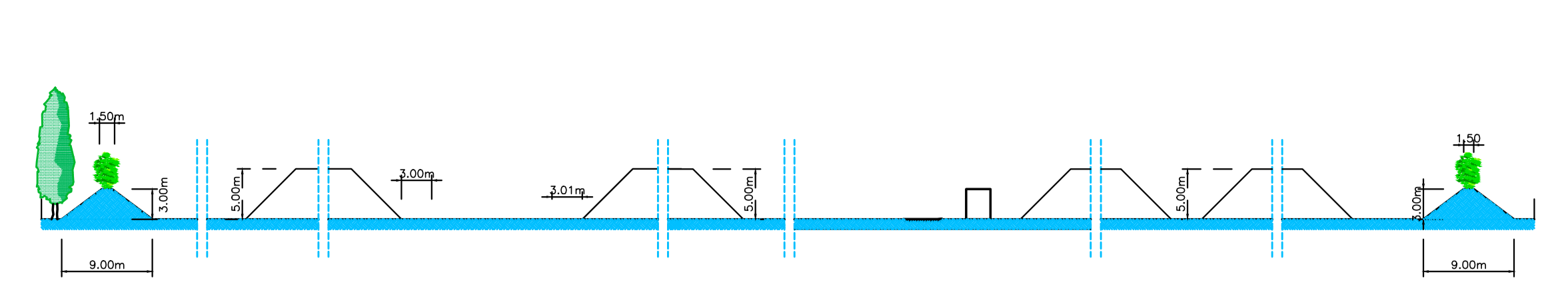
SEZIONE TIPO A-A' scala 1:500
