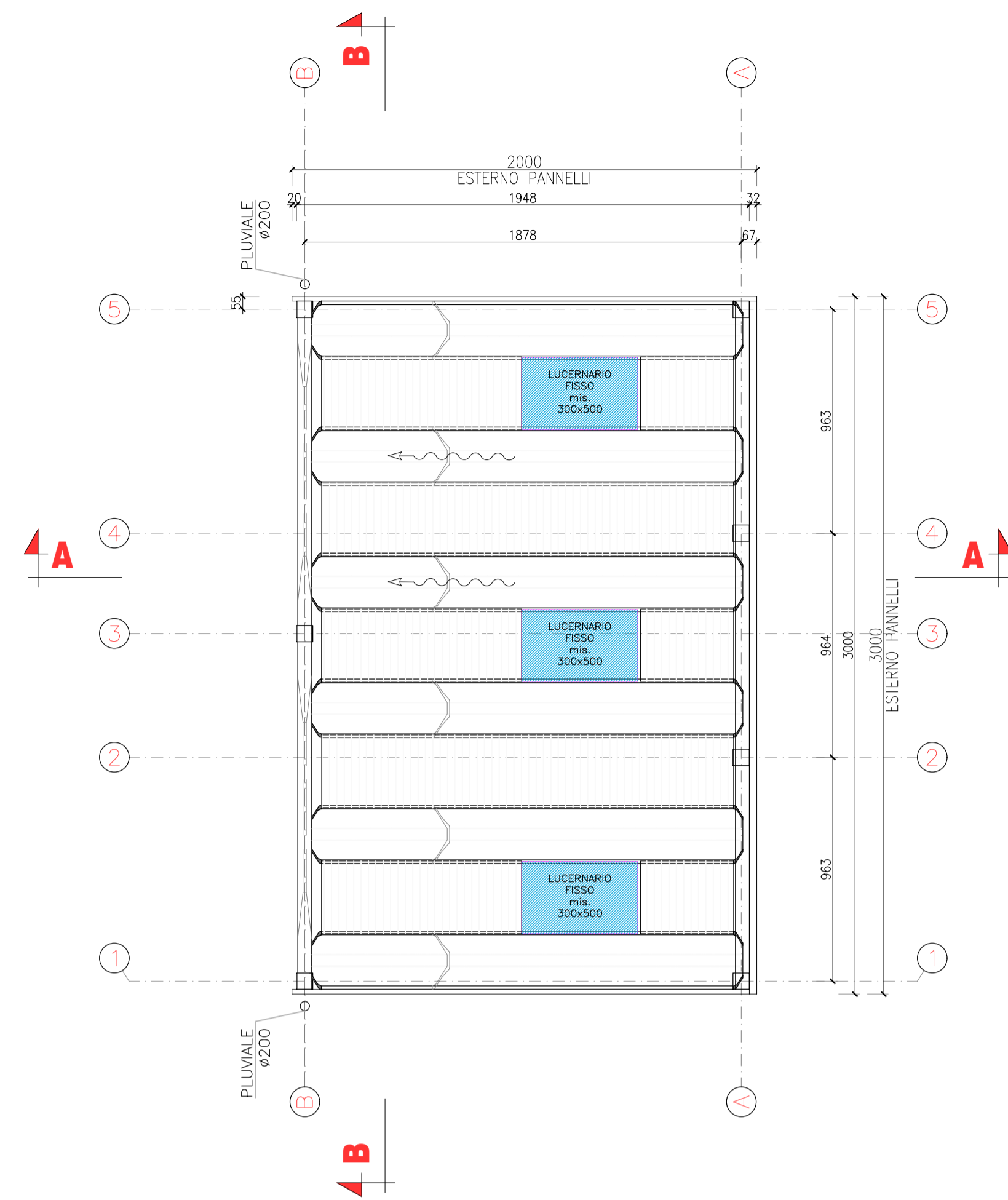
PIANTA COPERTURA
