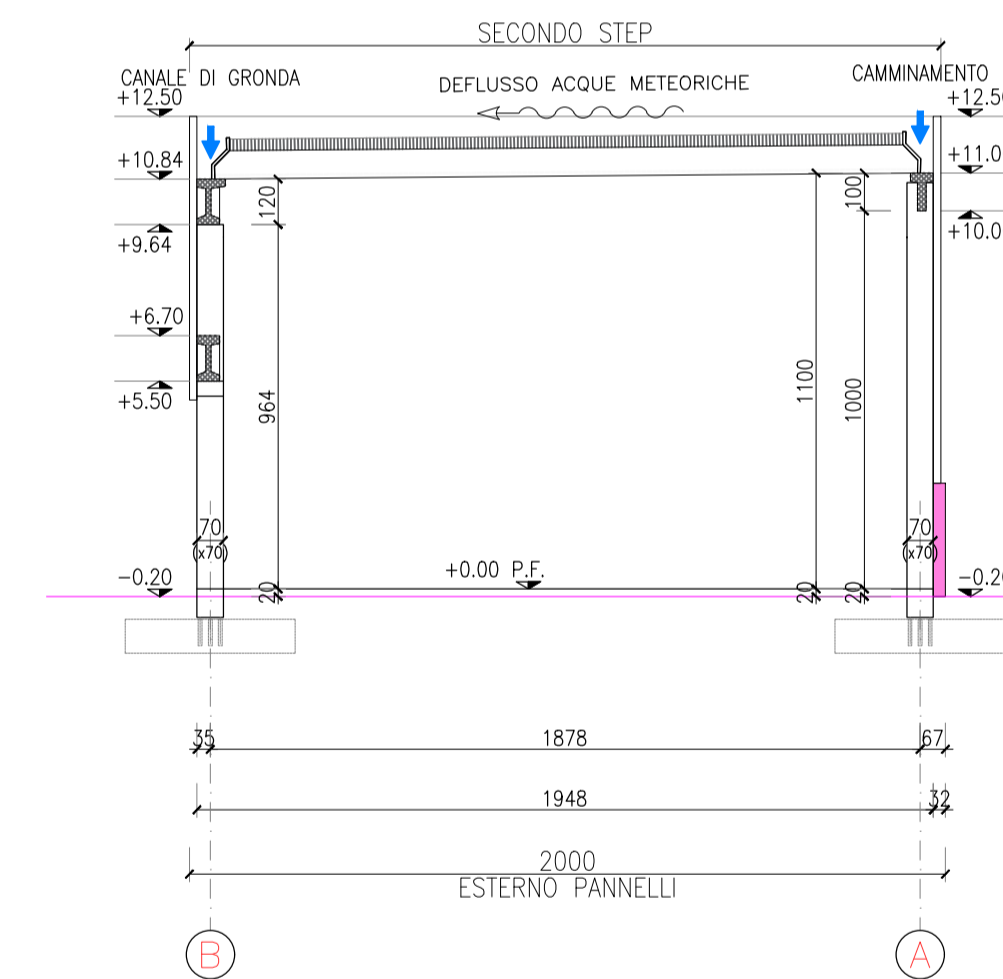
SEZIONE A-A
