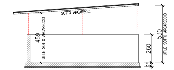
SEZIONE TIPO
