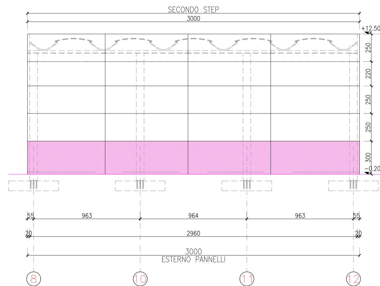
PROSPETTO SUD
