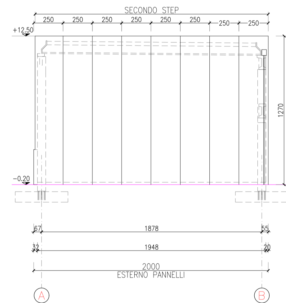
PROSPETTO EST
