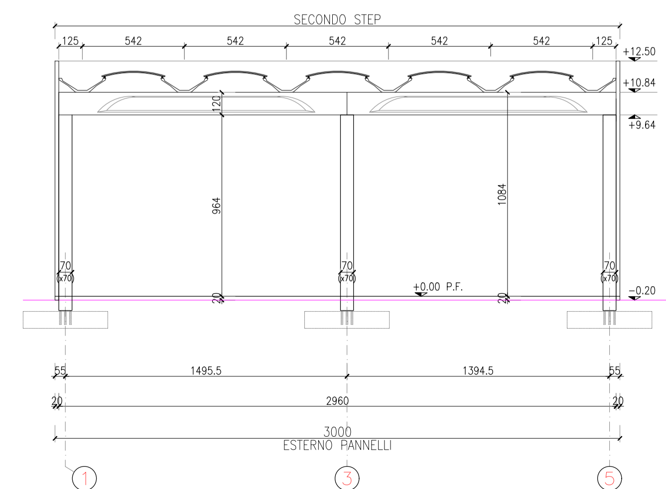
SEZIONE B-B
