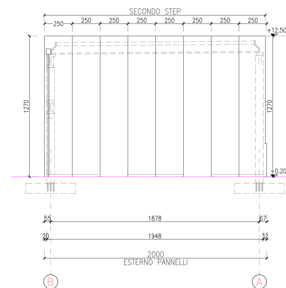
PROSPETTO OVEST
