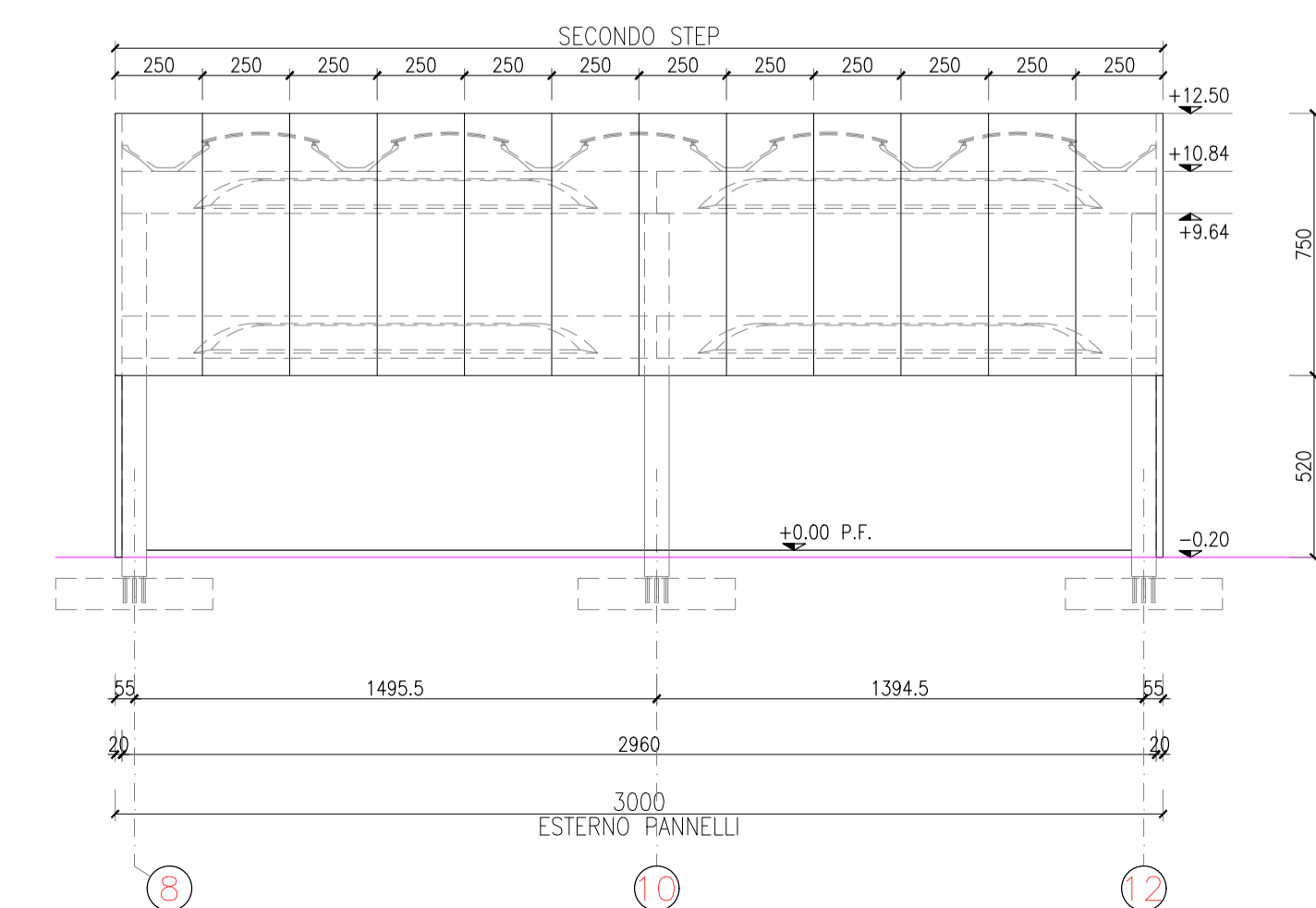
PROSPETTO NORD
