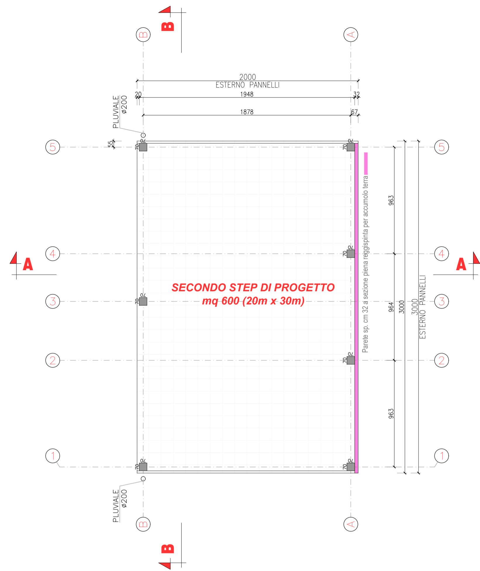
PIANTA PILASTRI
