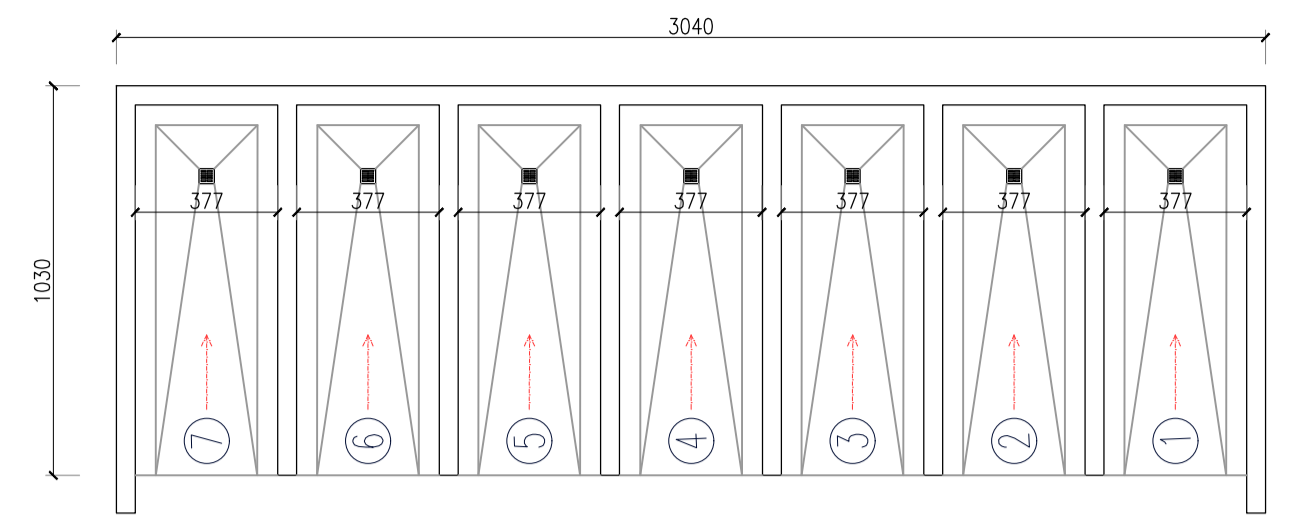
PIANTA 2° STEP - BOX STOCCAGGIO RIFIUTI
