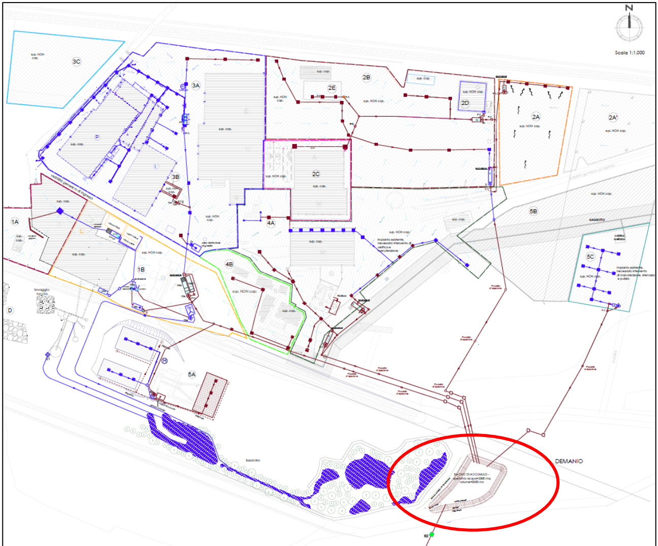
Figura 2.1. Area di utilizzo terre da scavo per realizzazione arginello bacino di contenimento
