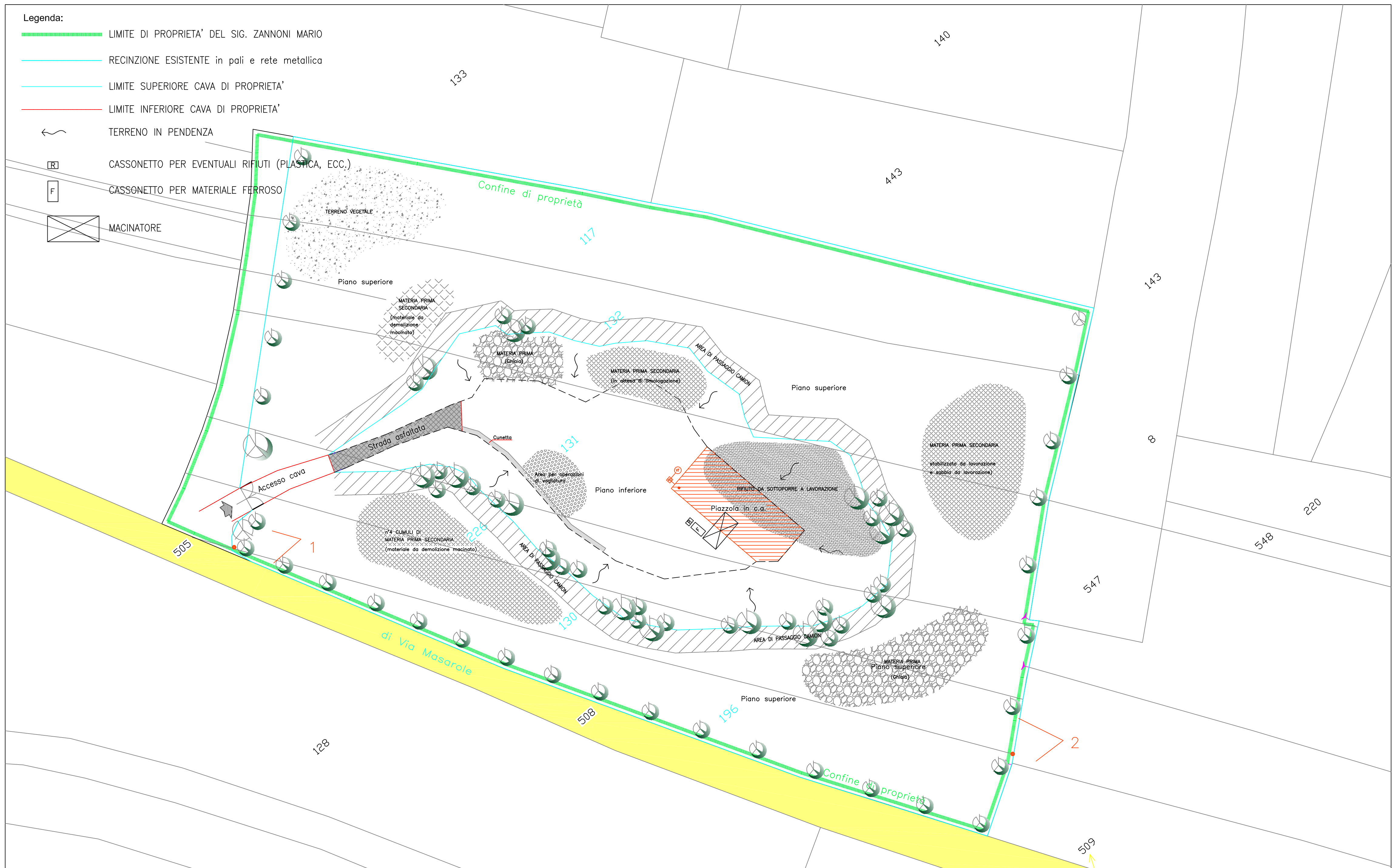
PLANIMETRIA Scala 1:500
