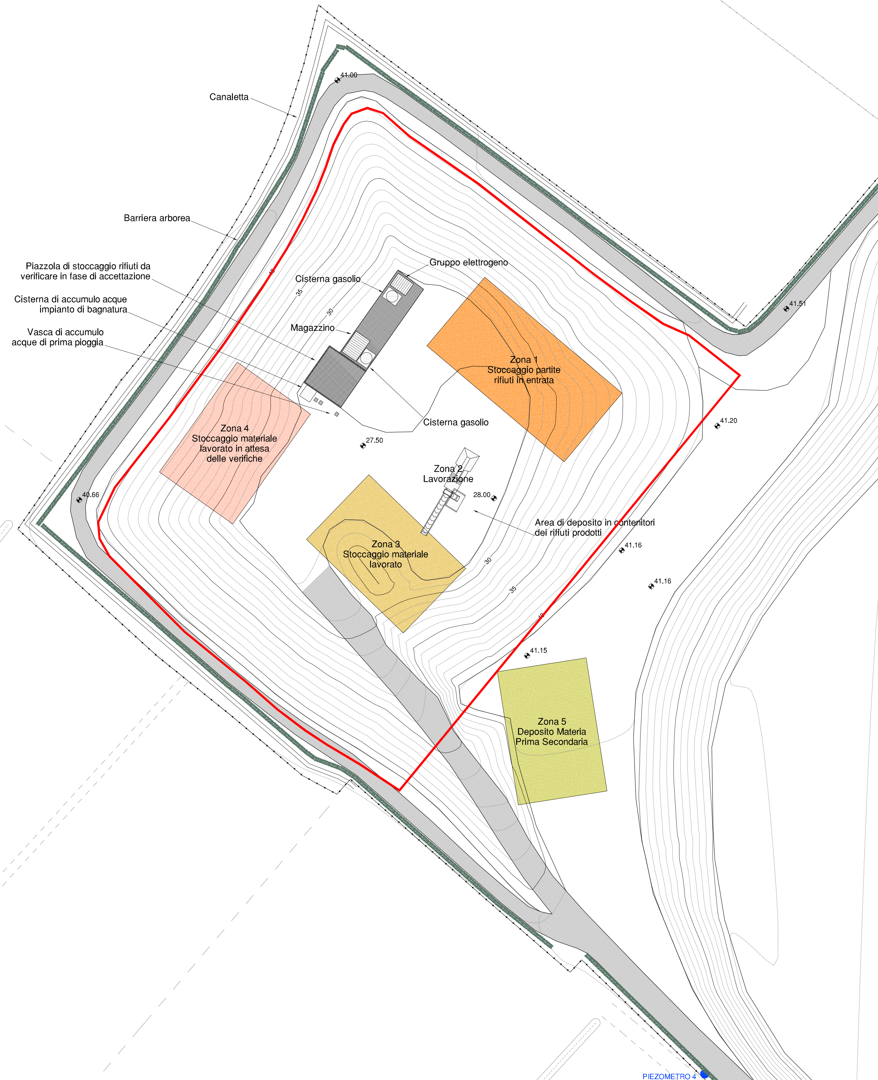
STATO AUTORIZZATO - Scala 1:500
