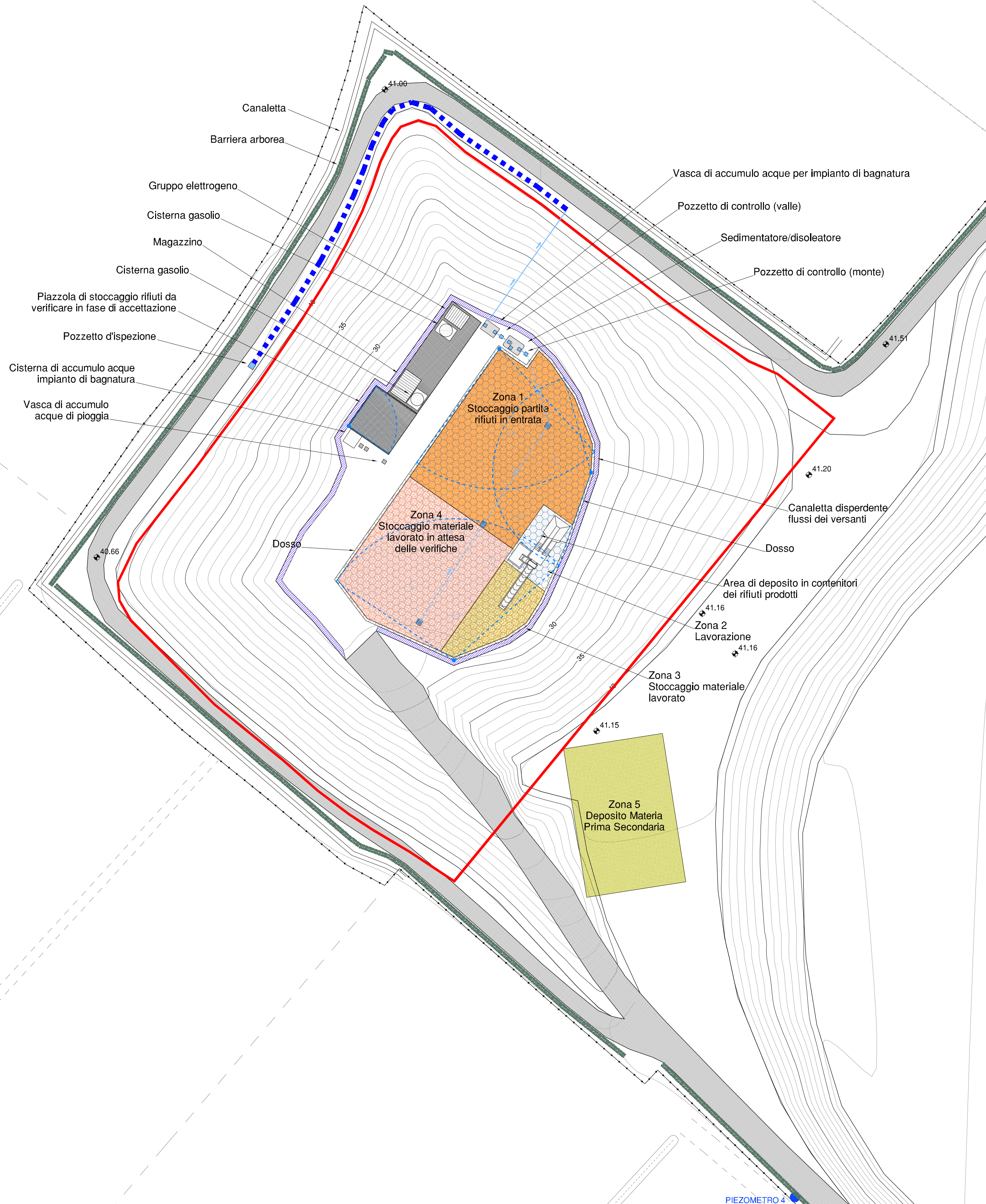
STATO ADEGUATO - Scala 1:500
