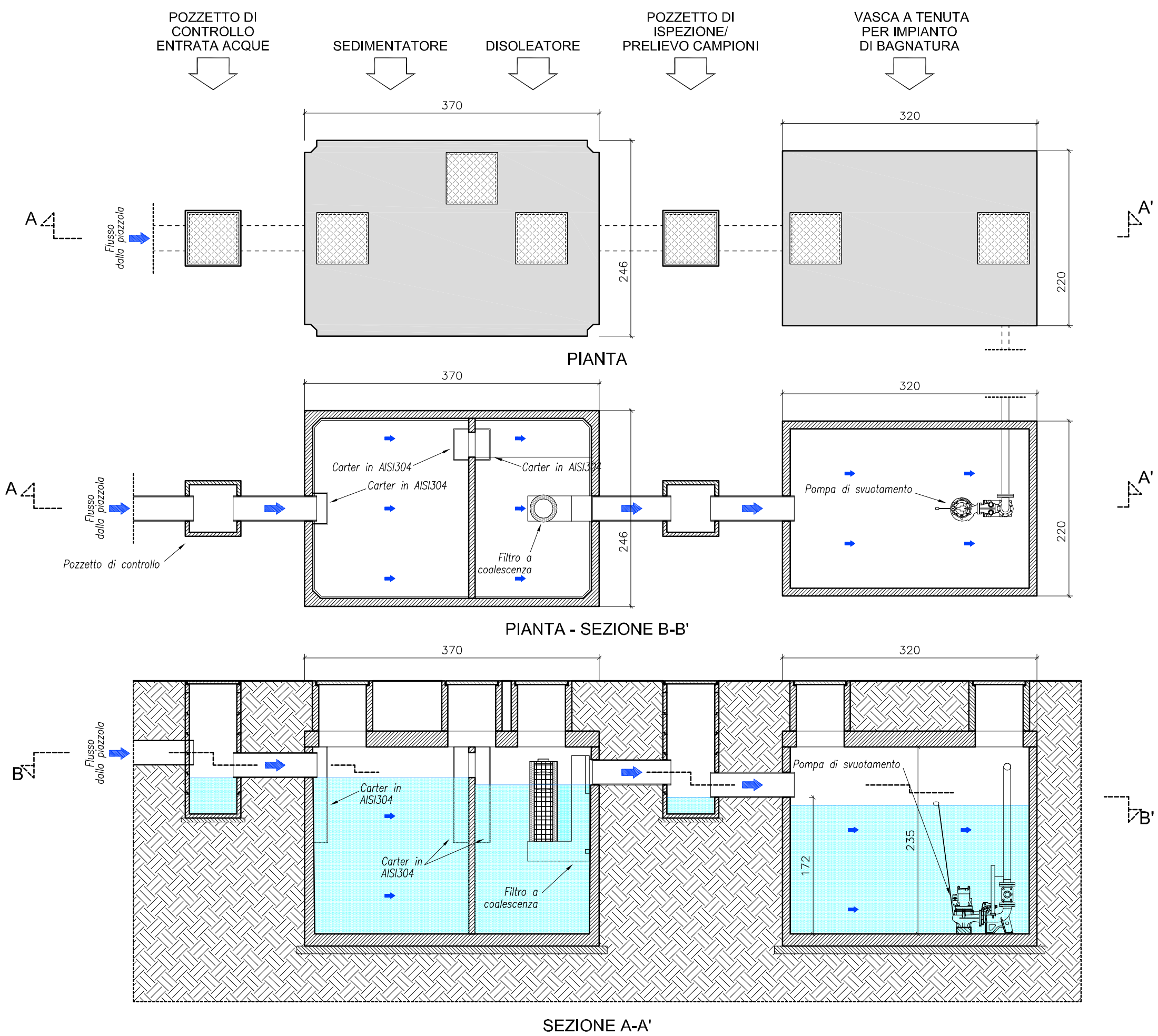
SEDIMENTATORE - DISOLEATORE - VASCA DI ACCUMULO - Scala 1:50
