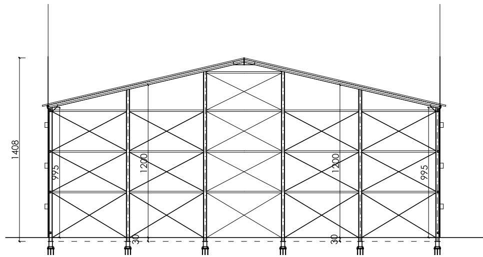
CAPANNONE 2-3 - SEZIONE (baraccatura) scala 1:50
