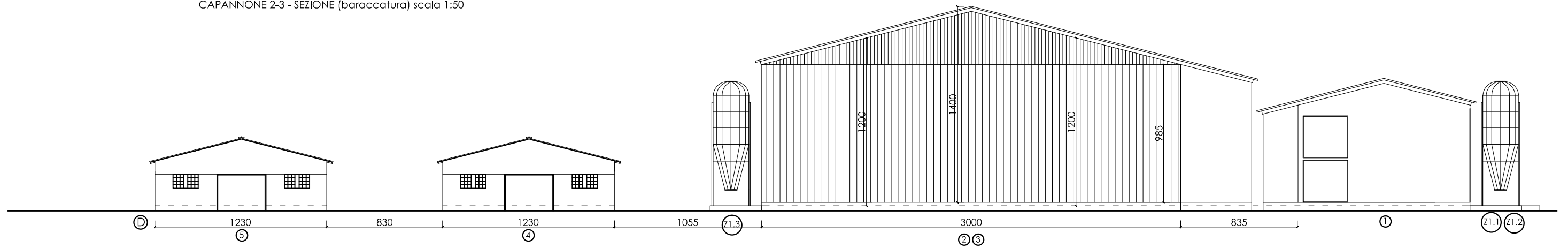
CAPANNONE 2-3 - SEZIONE (baraccatura) scala 1:50
