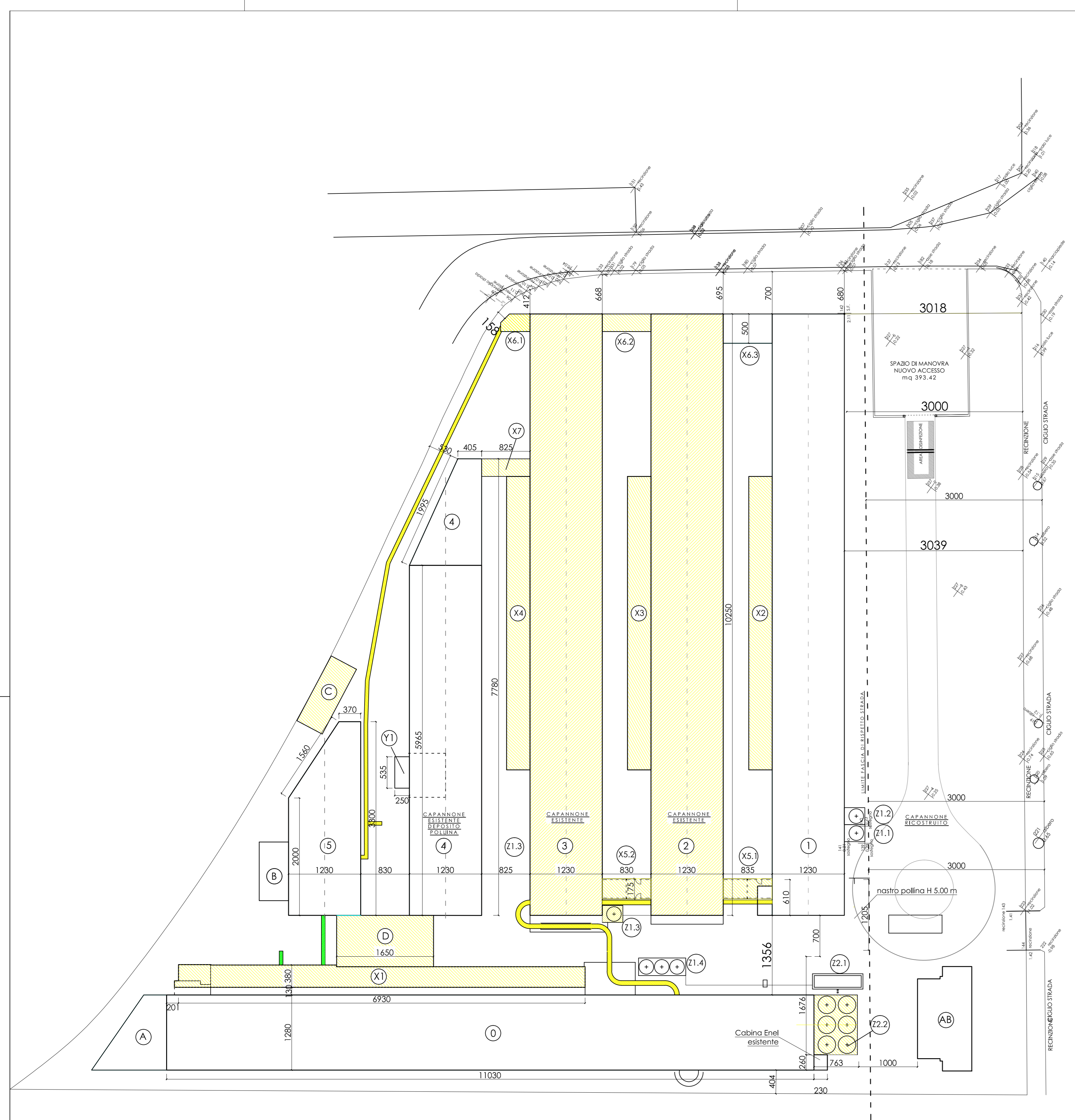
STATO APPROVATO PdC 077 del 04.05.2016 DEMOLIZIONI / VOLUMI NON REALIZZATI
