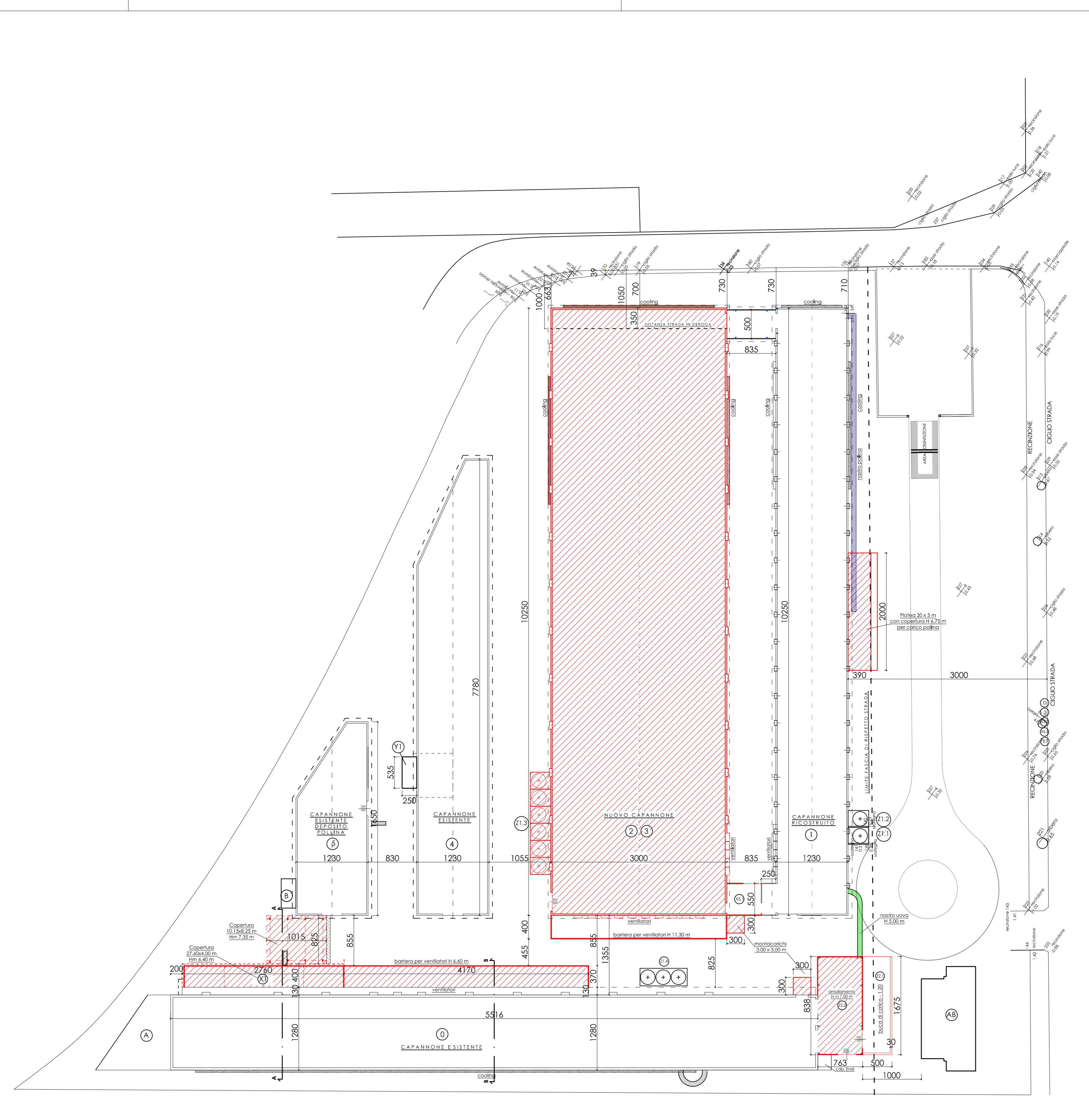
STATO DI PROGETTO - VARIANTE COSTRUZIONI / ACCORPAMENTO VOLUMI
