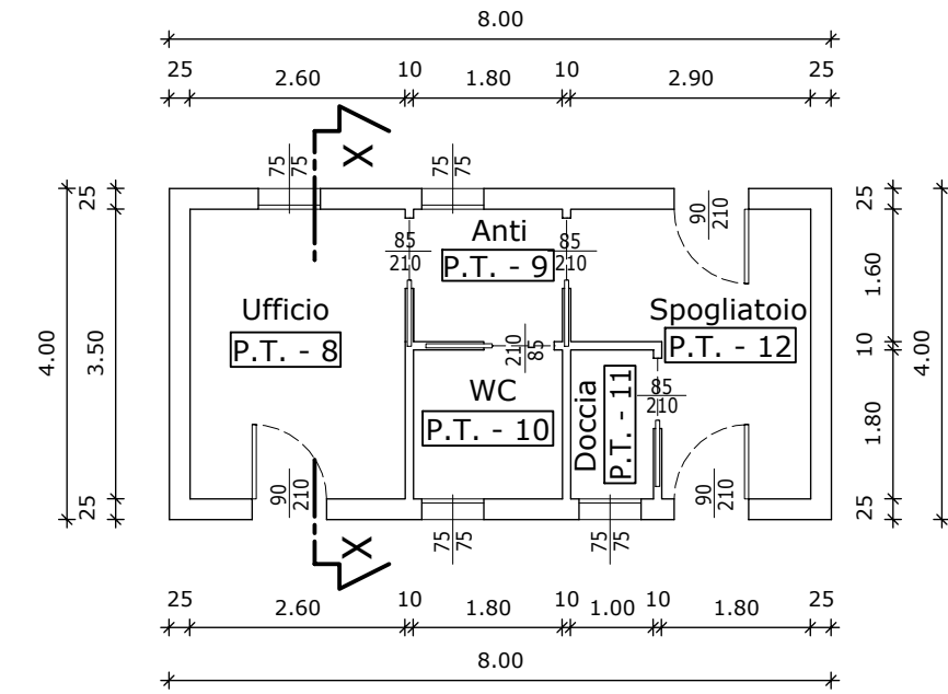
PIANTA ZONA FILTRO
