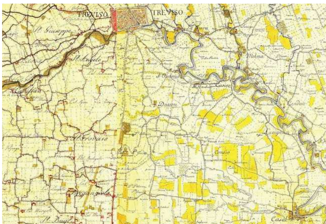
Figura 4-11- Anton von Zach, Carta militare topografico-geometrica del Ducato di Venezia, 1805
