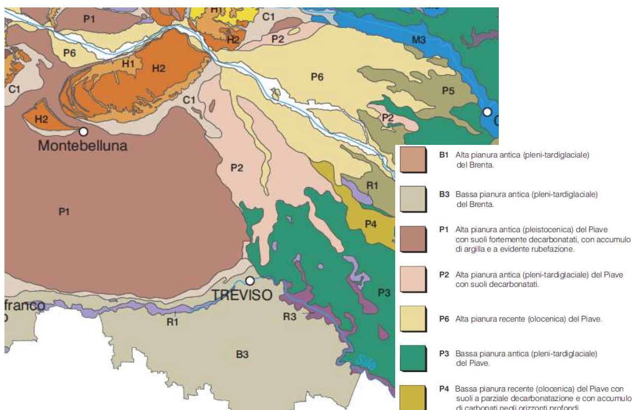
Figura 4-4- Stralcio Carta dei suoli – Provincia di Treviso – fonte: ARPAV
