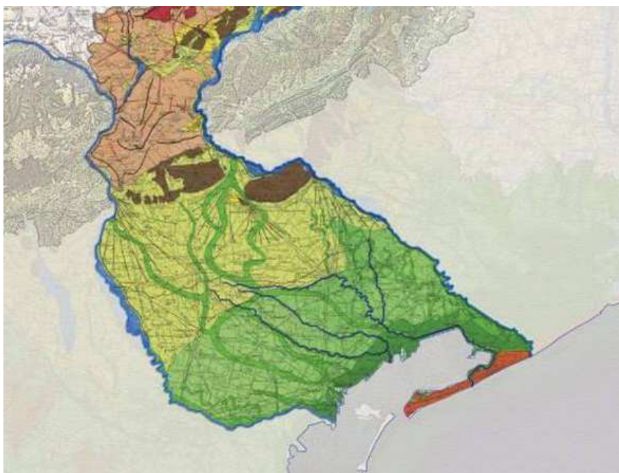
Figura 4-3- Carta geologica Regione Veneto
