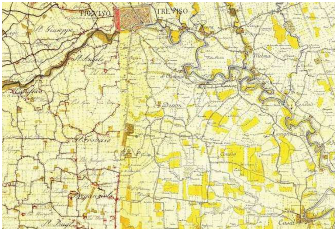
Figura 4-7- Anton von Zach, Carta militare topografico-geometrica del Ducato di Venezia, 1805
