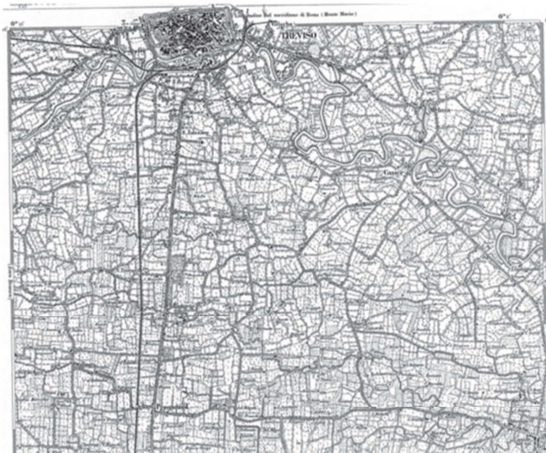
Figura 4-12- Carta militare IGM 1887
