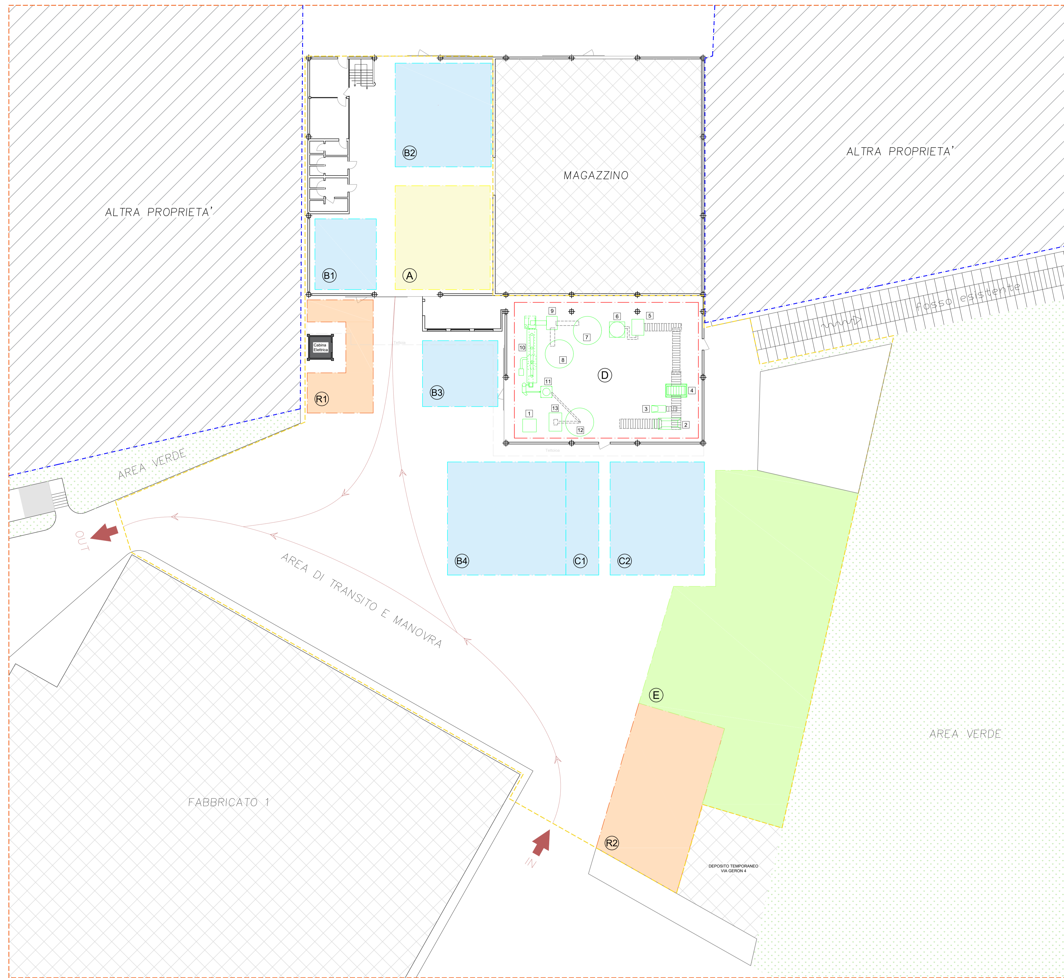
PARTICOLARE AREA IMPIANTO DI RECUPERO - Scala 1:200
