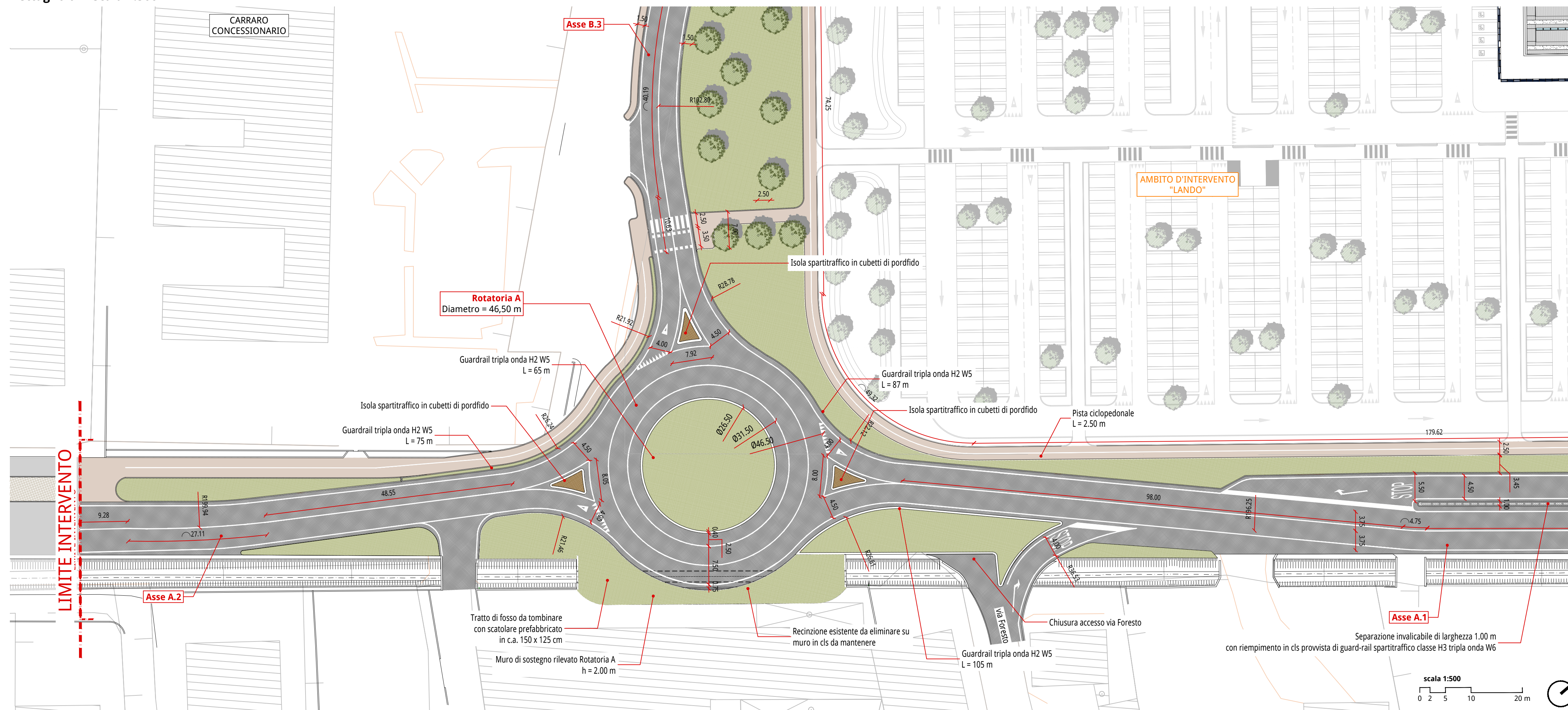
Dettaglio 01 - scala 1:500
