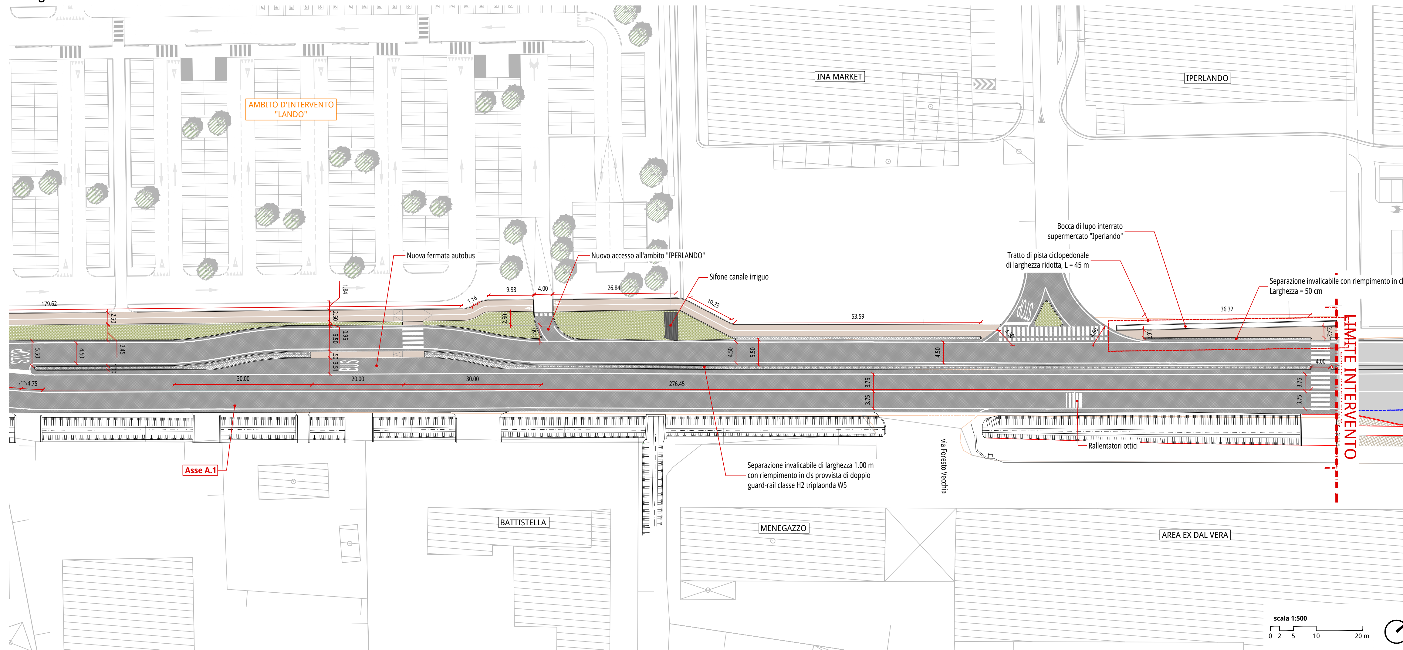
Dettaglio 01 - scala 1:500
