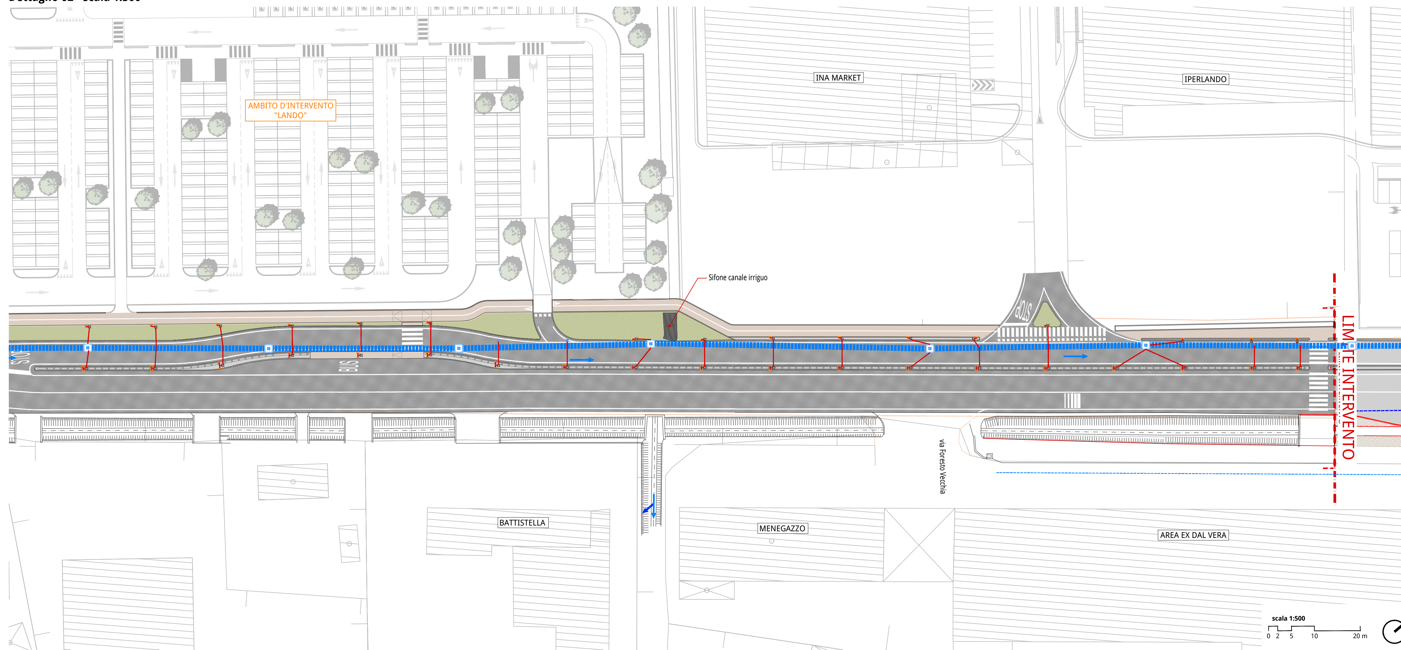
Dettaglio 01 - scala 1:500
