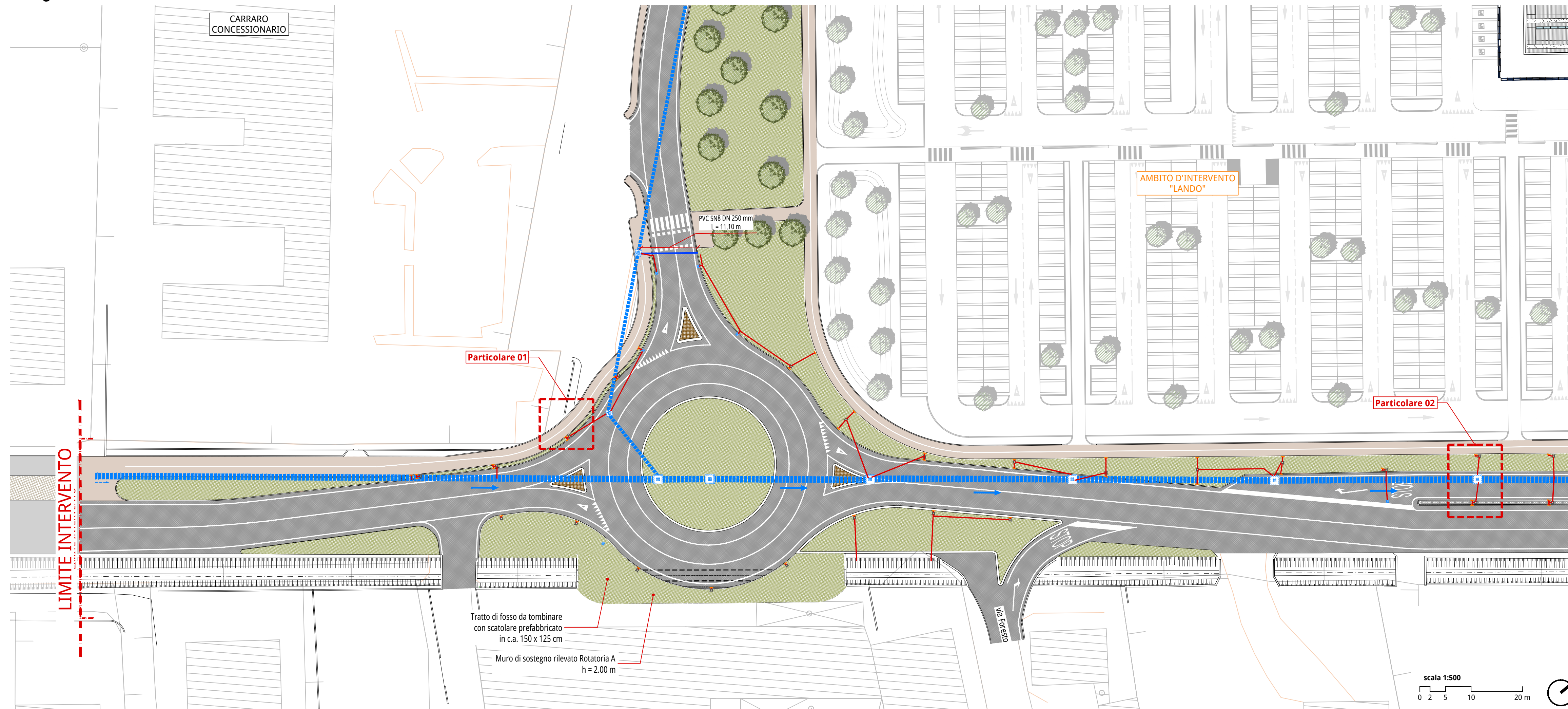
Dettaglio 01 - scala 1:500
