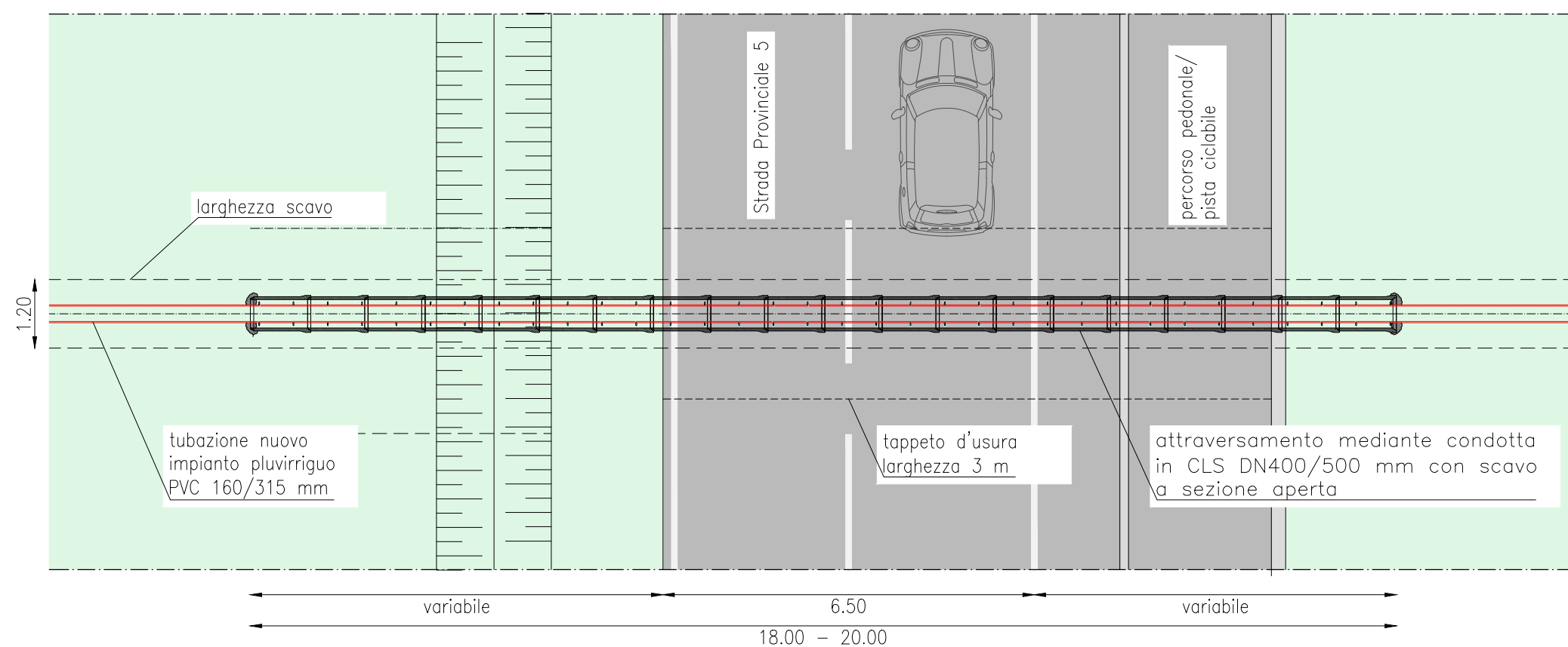
SEZIONE TIPO DI POSA TUBOGUAINA PVC 315 mm scala 1:20
