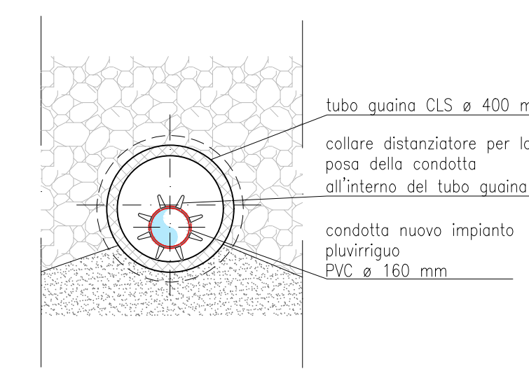
SEZIONE TIPO TUBOGUAINA PVC 160 mm scala 1:20
