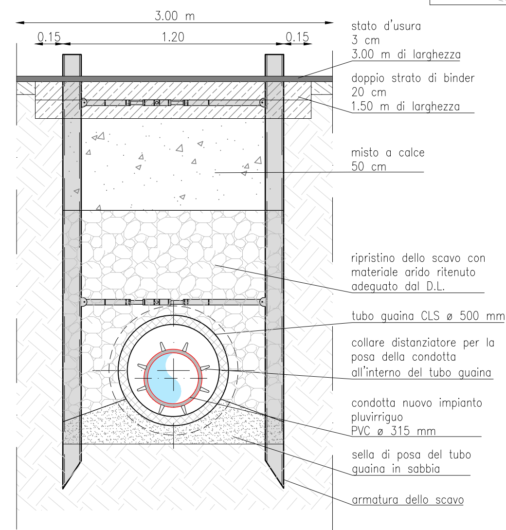
SEZIONE TIPO DI POSA TUBOGUAINA PVC 315 mm scala 1:20
