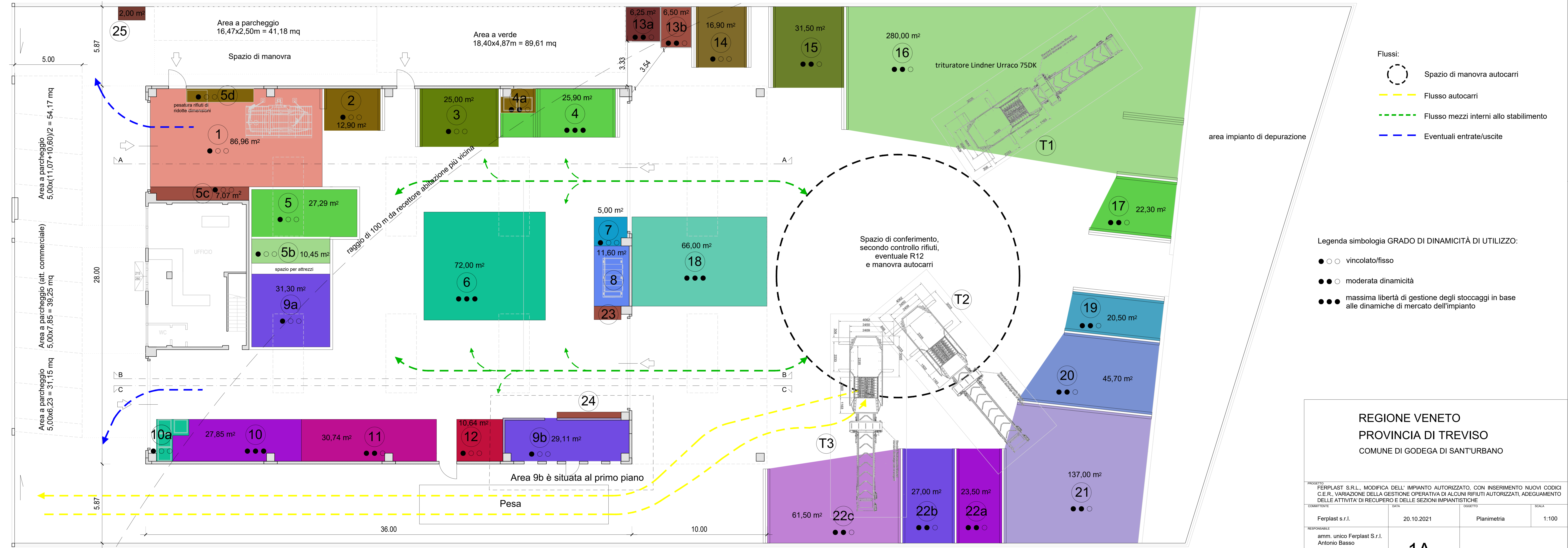
T1-T2-T3 Posizioni indicative del trituratore mobile in attività
