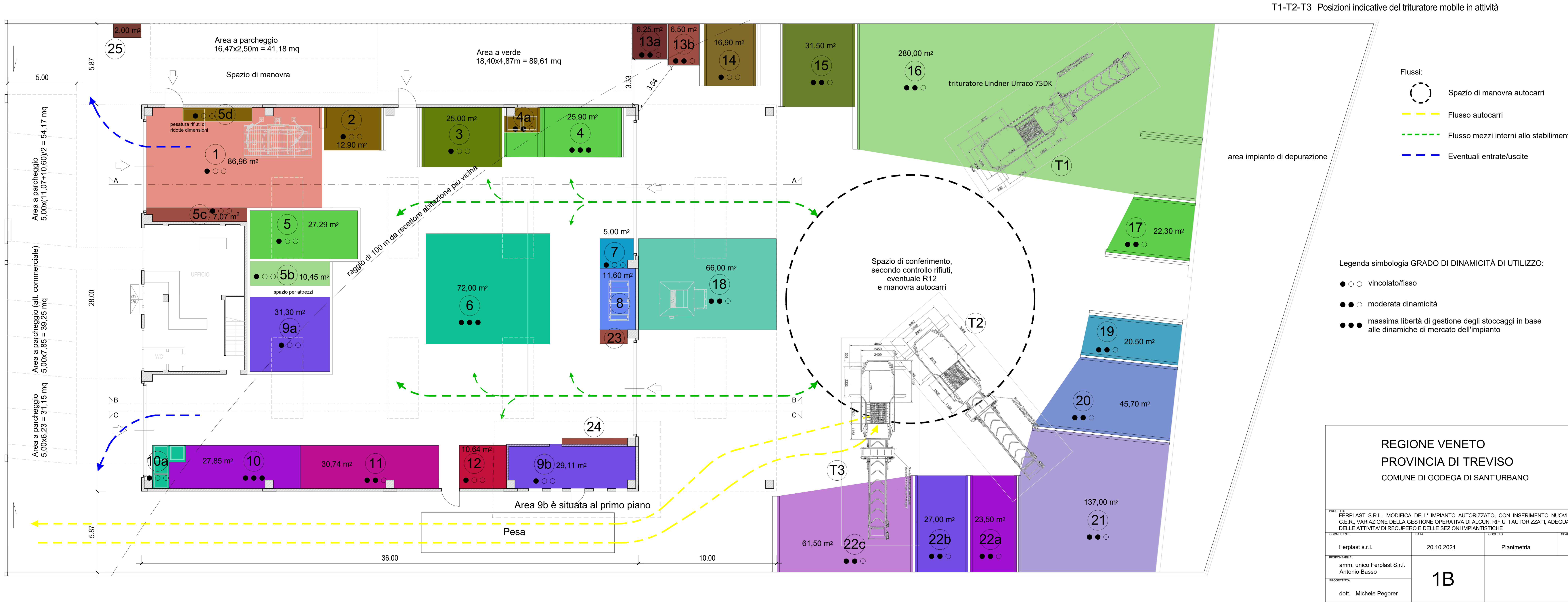
T1-T2-T3 Posizioni indicative del tritratore mobile in attività
