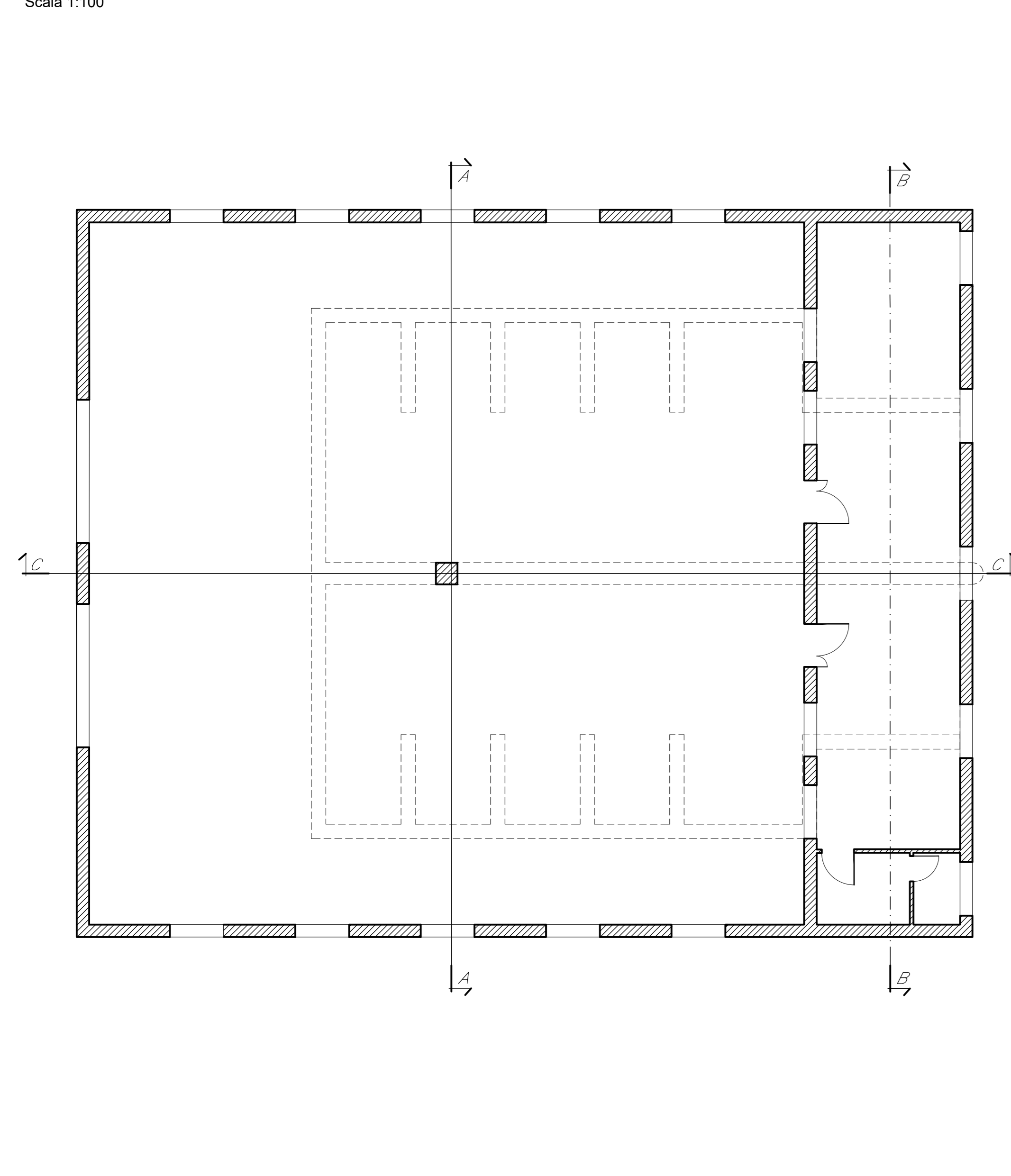
Piante Edificio e Vasca Scala 1:100
