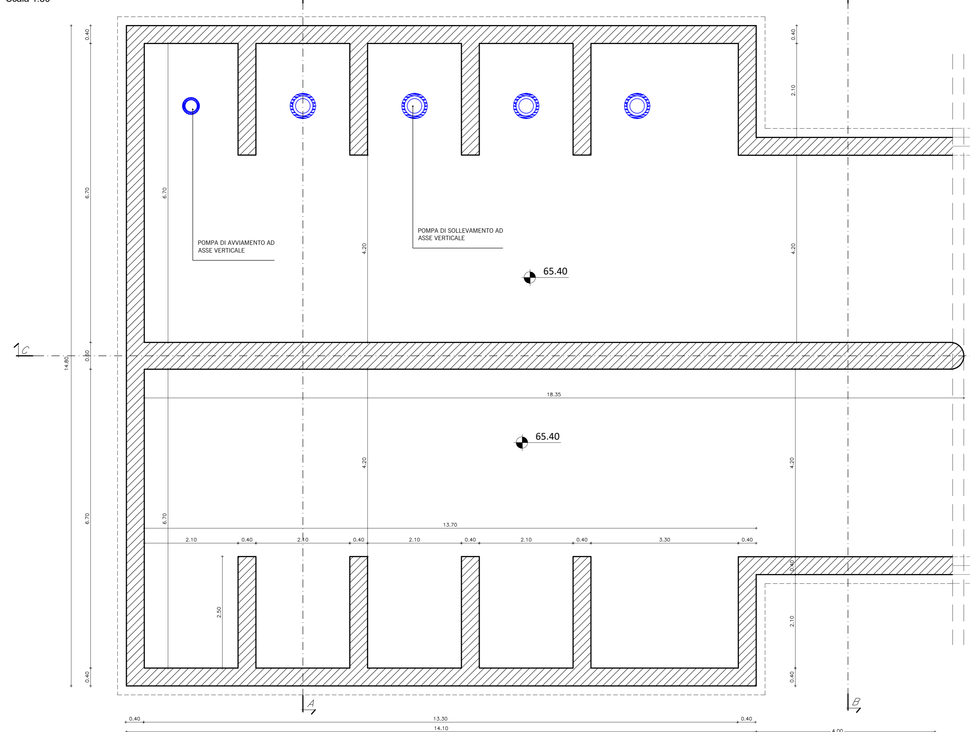
Sezione D-D - Pianta Vasca Scala 1:50
