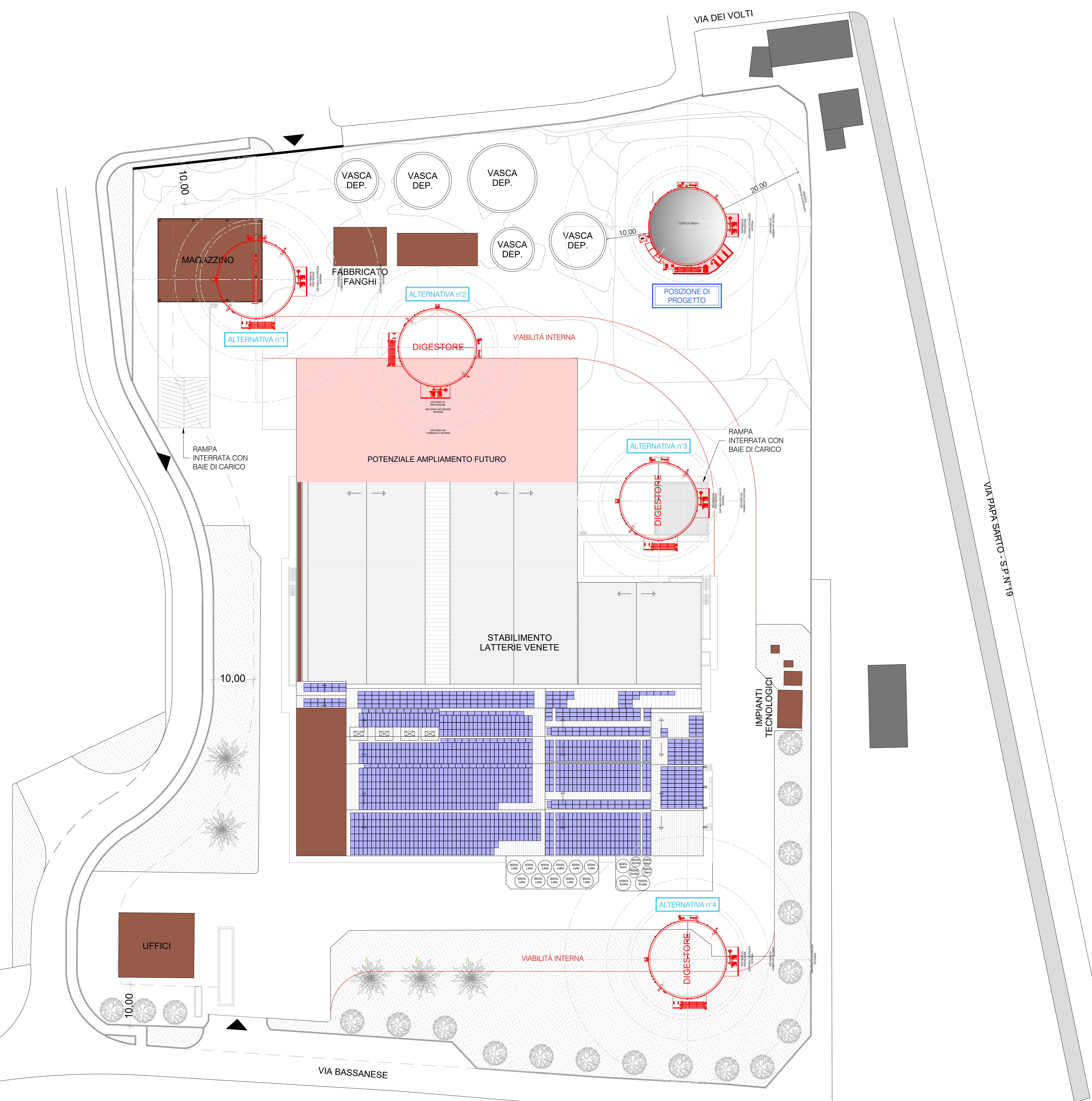
PLANIMETRIA GENERALE con schema rete fognaria Scala 1:500
