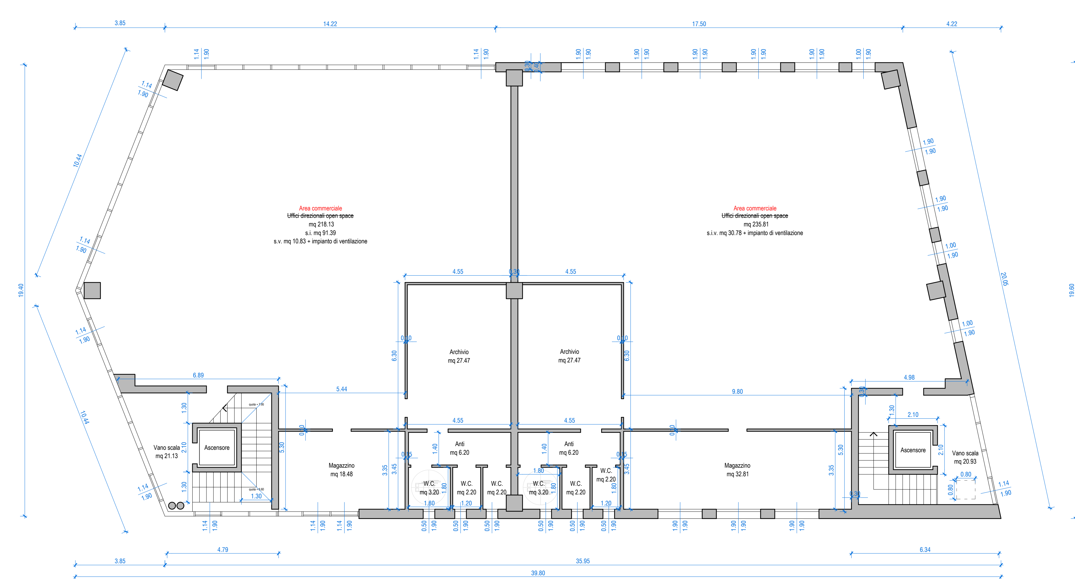
PIANO PRIMO Stato di progetto
