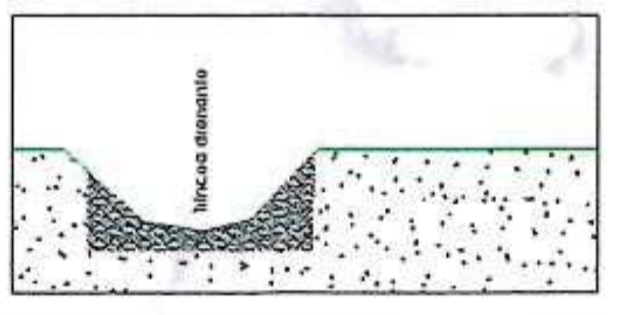
Sezione Tipo y-y scala 1:50 particolare trincea drenante
