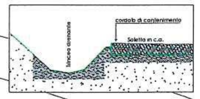
Sezione Tipo x-x scala 1:50 particolare soletta a ridosso della trincea
