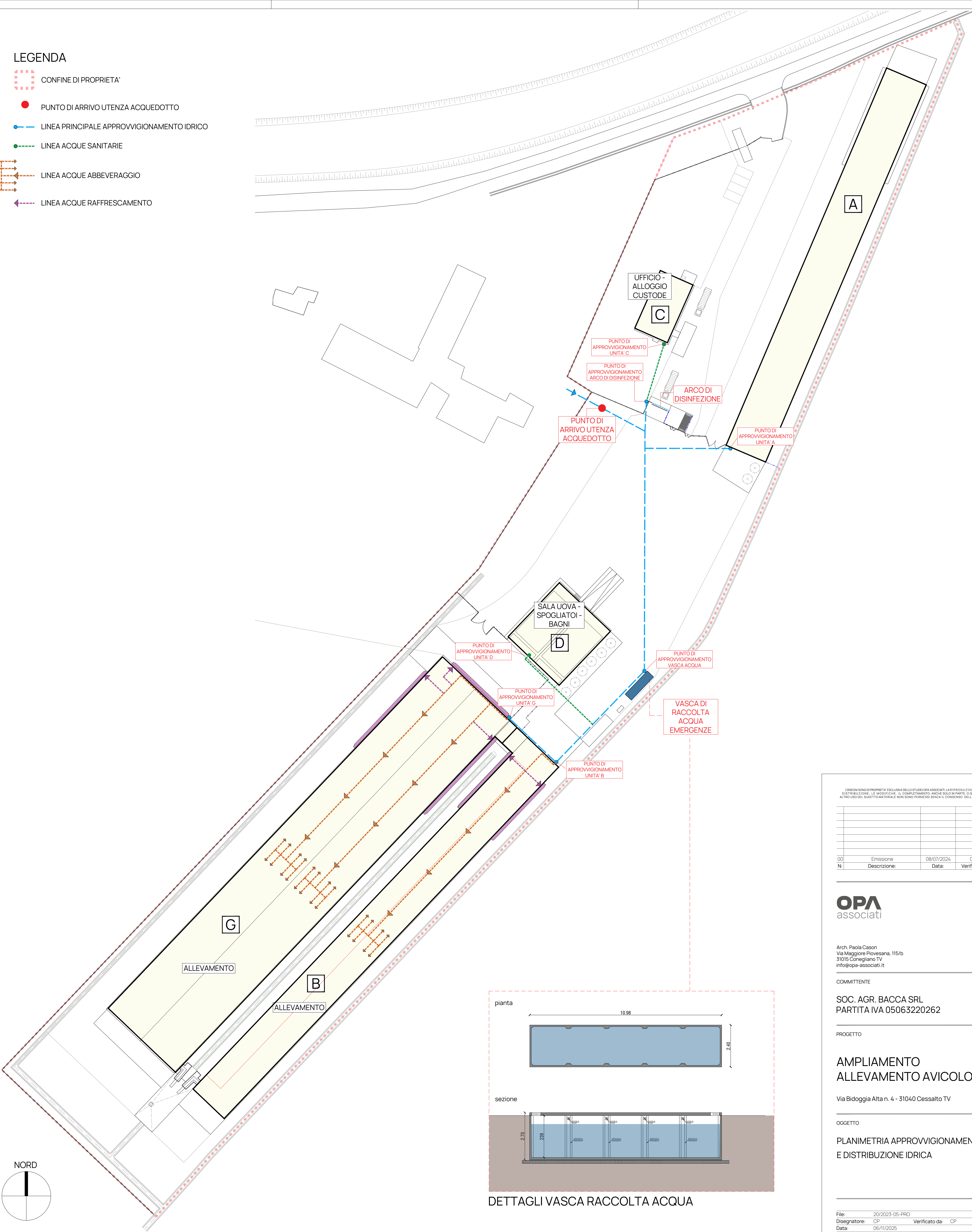
PLANIMETRIA GENERALE SCALA 1:500
