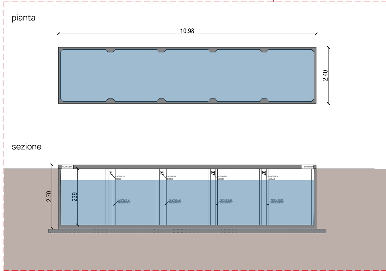
DETTAGLI VASCA RACCOLTA ACQUA
