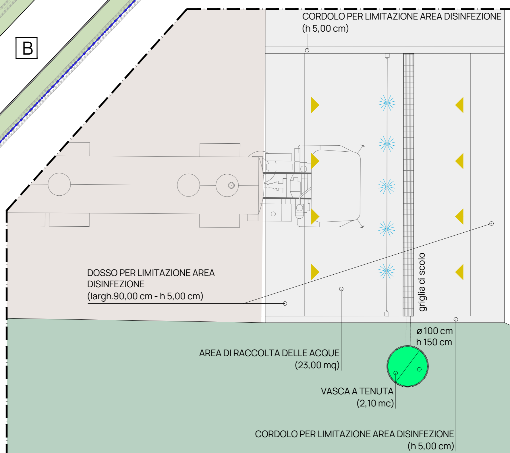
R03 AREA ARCO DI DISINFEZIONE AUTOMEZZI SCALA 1:50
