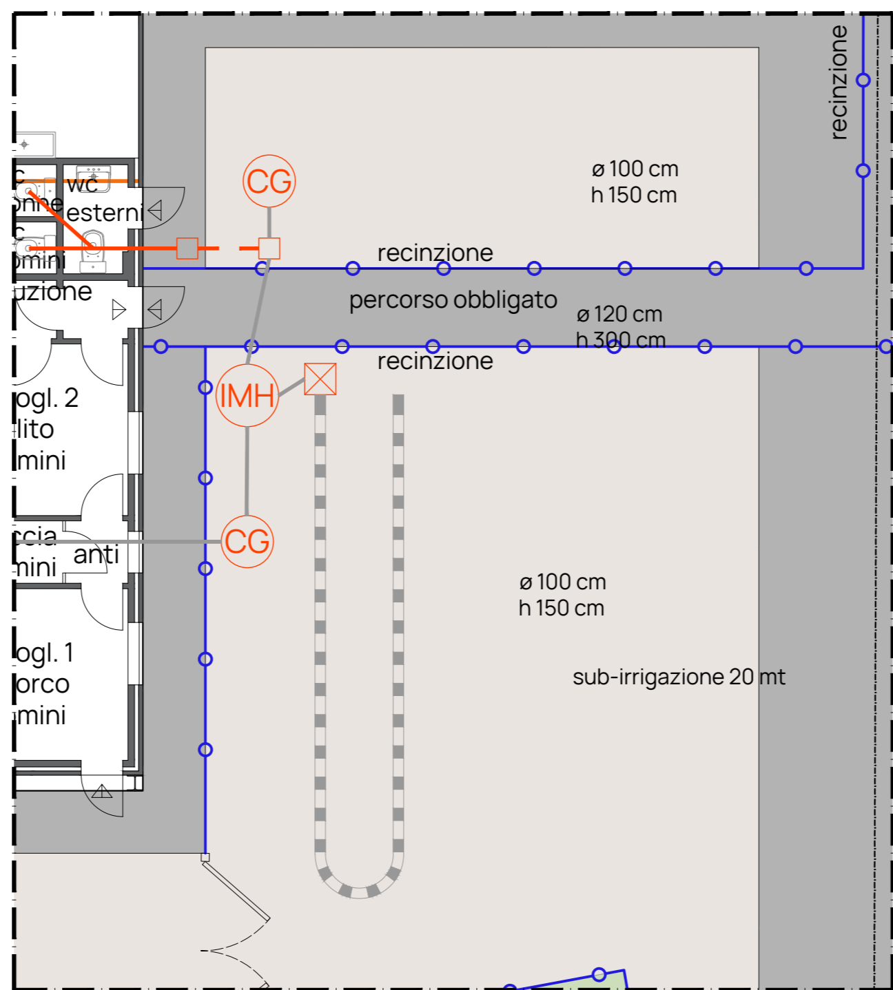
R02 SCARICHI SPOGLIATOI SALA UOVA SCALA 1:100
