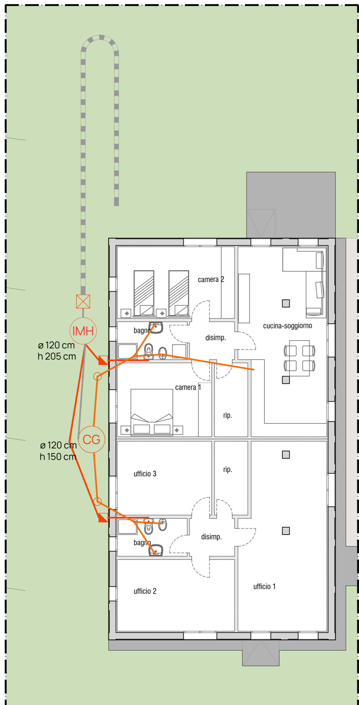
R01 SCARICHI UFFICI / ALLOGGIO CUSTODE SCALA 1:100
