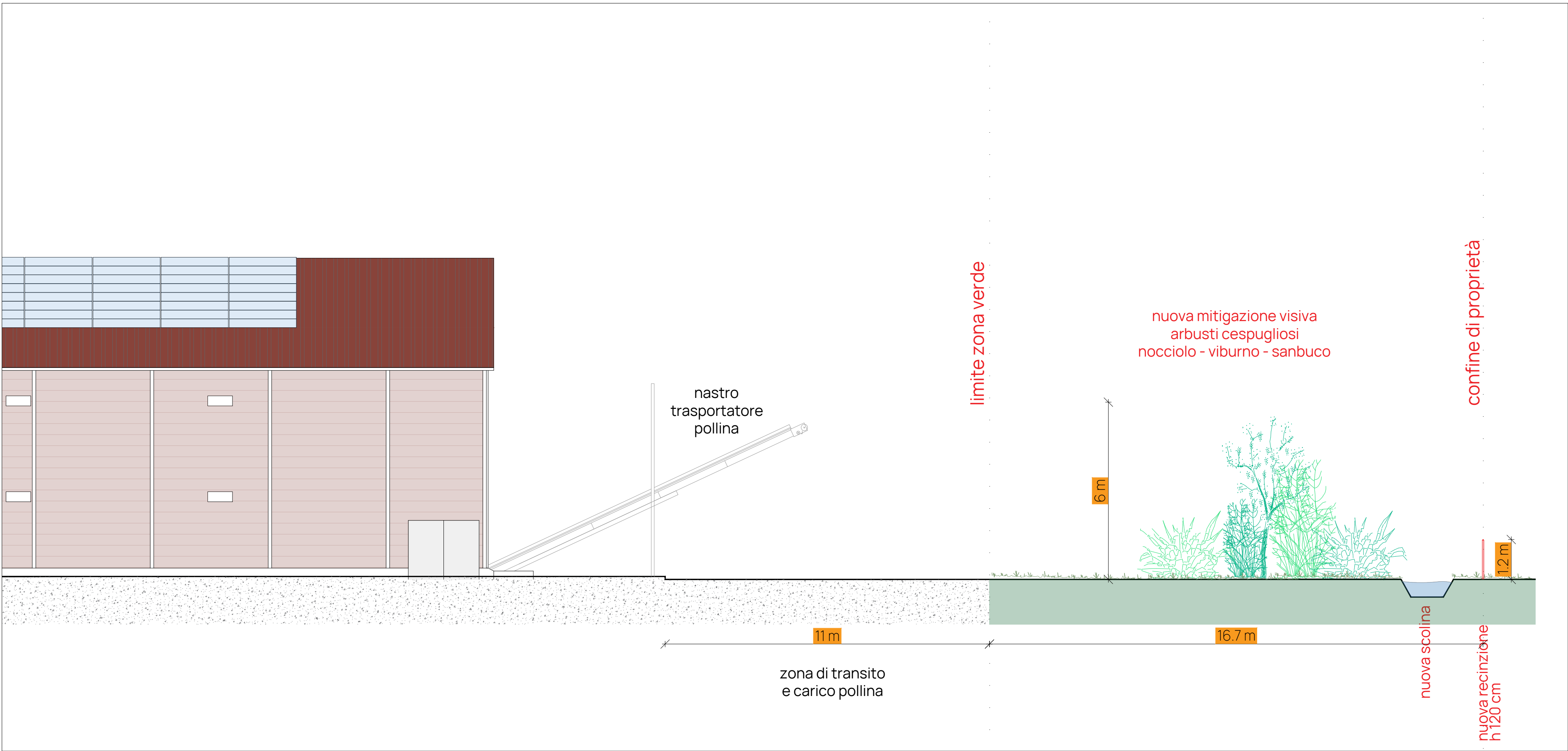
SEZIONE B - B
