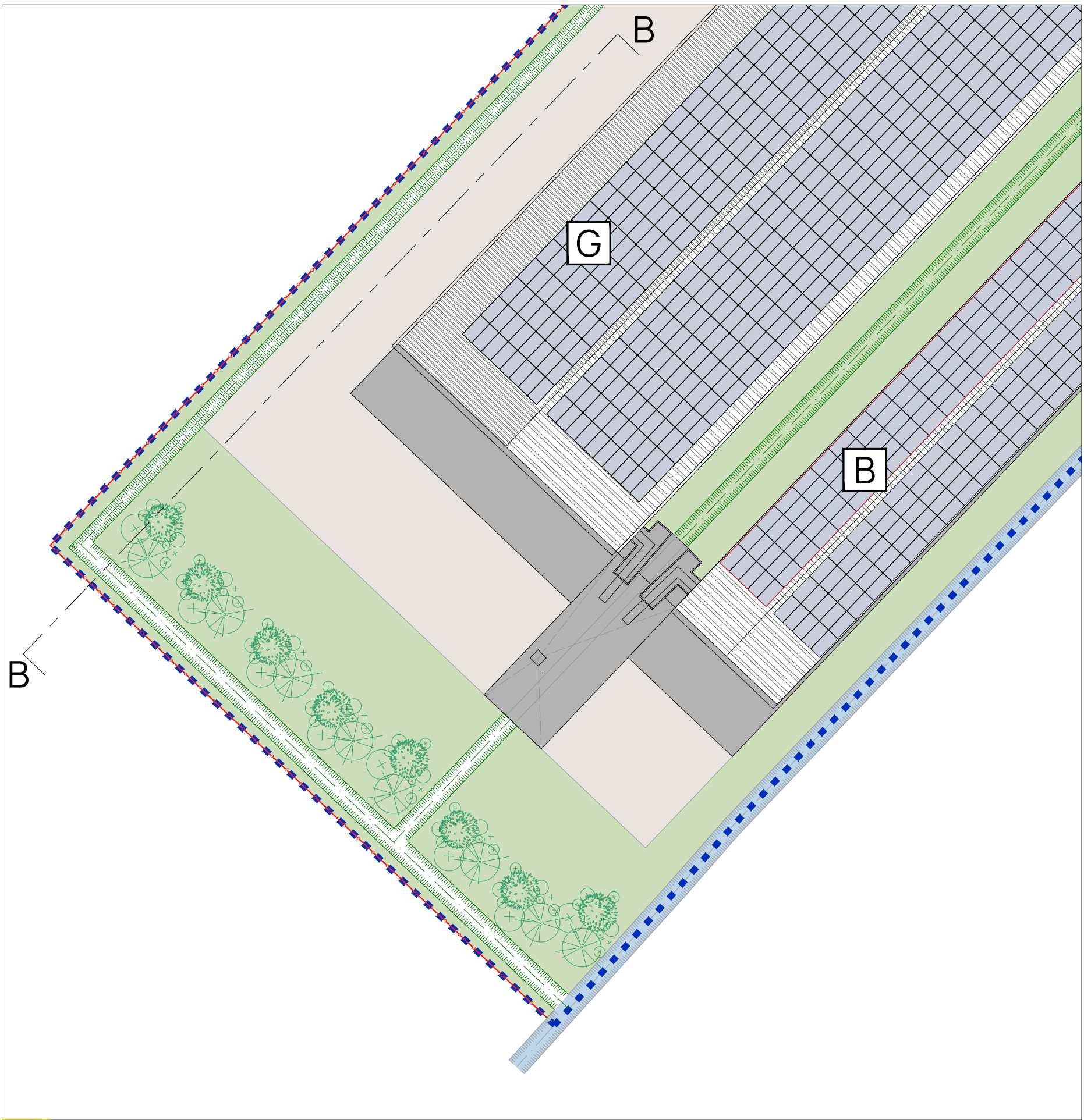
PARTICOLARE 2 - MITIGAZIONE CONFINE SUD
