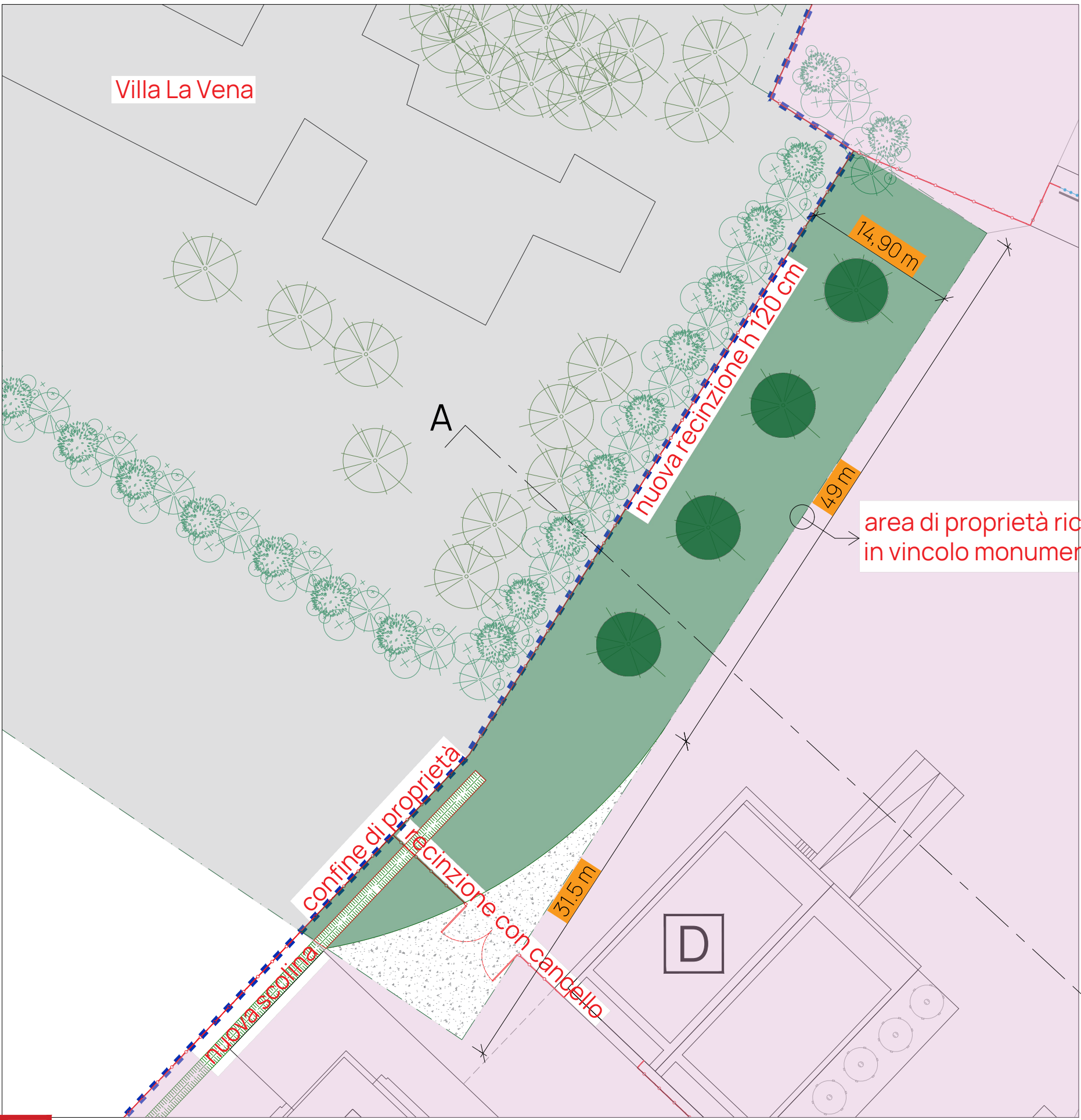
PARTICOLARE 1 - PORZIONE DI AREA RIENTRANTE NEL VINCOLO MONUMENTALE
