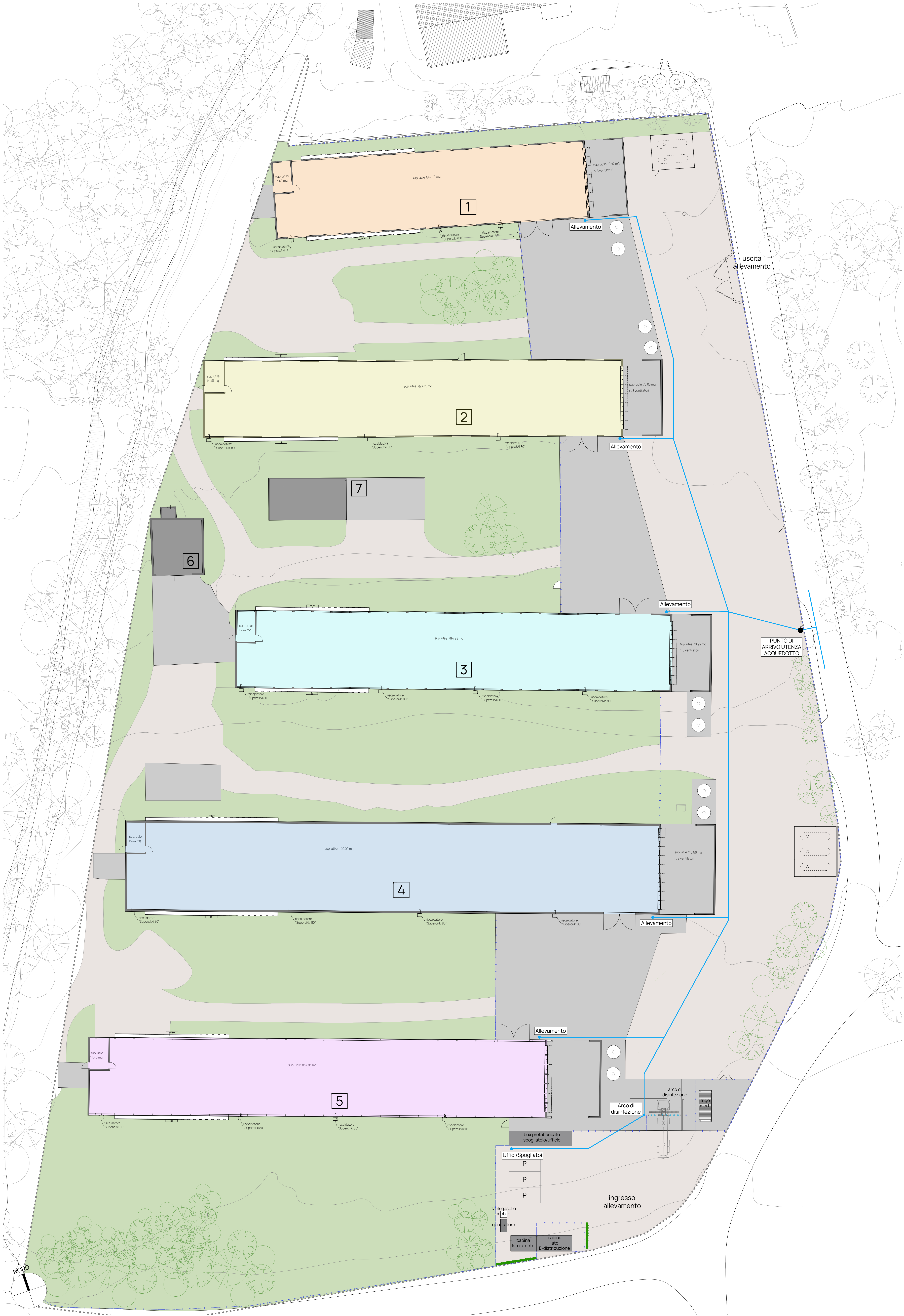
PLANIMETRIA GENERALE SCALA 1:200
