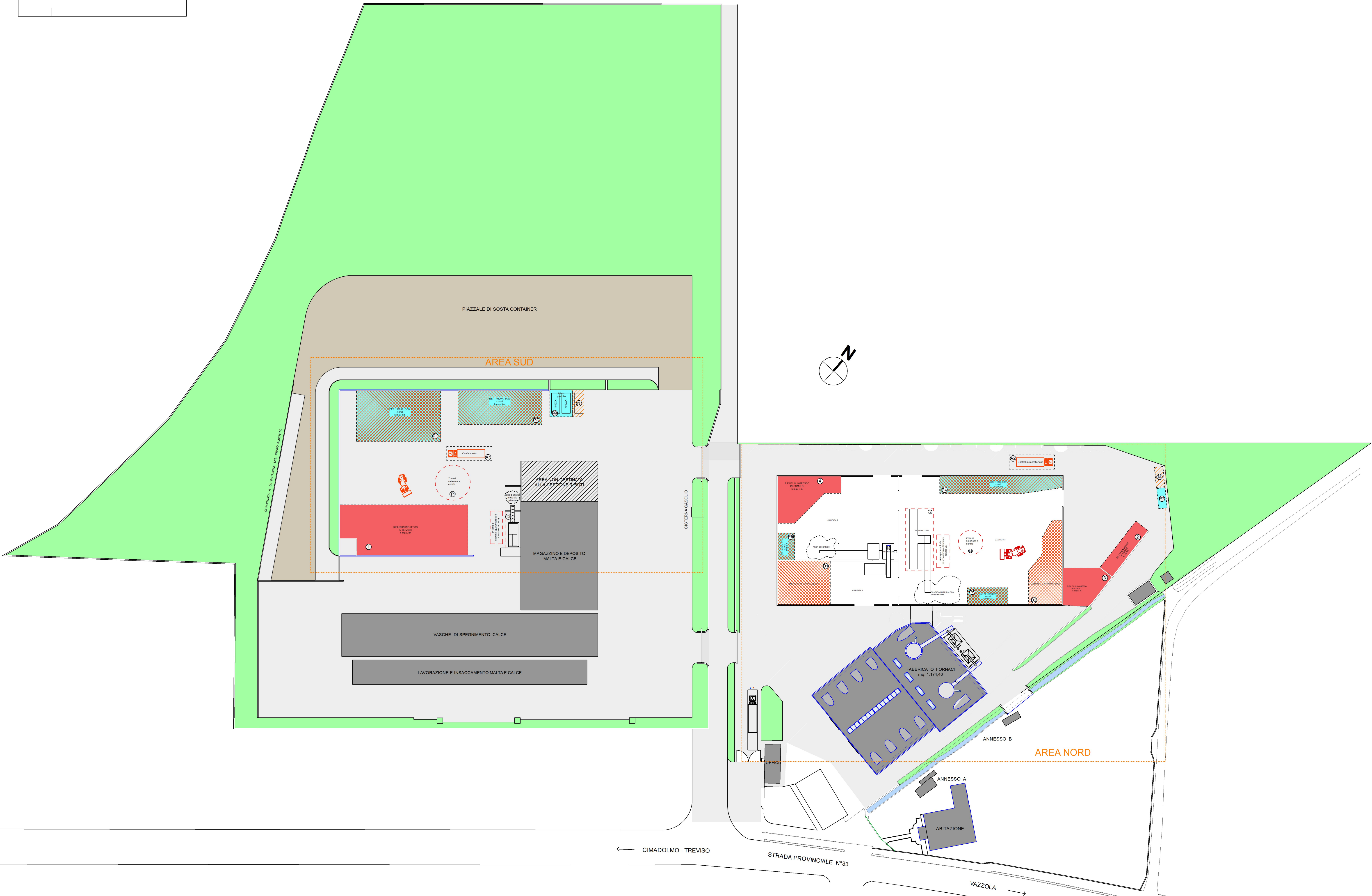
PLANIMETRIA GENERALE DELL'AZIENDA SC. 1:500
