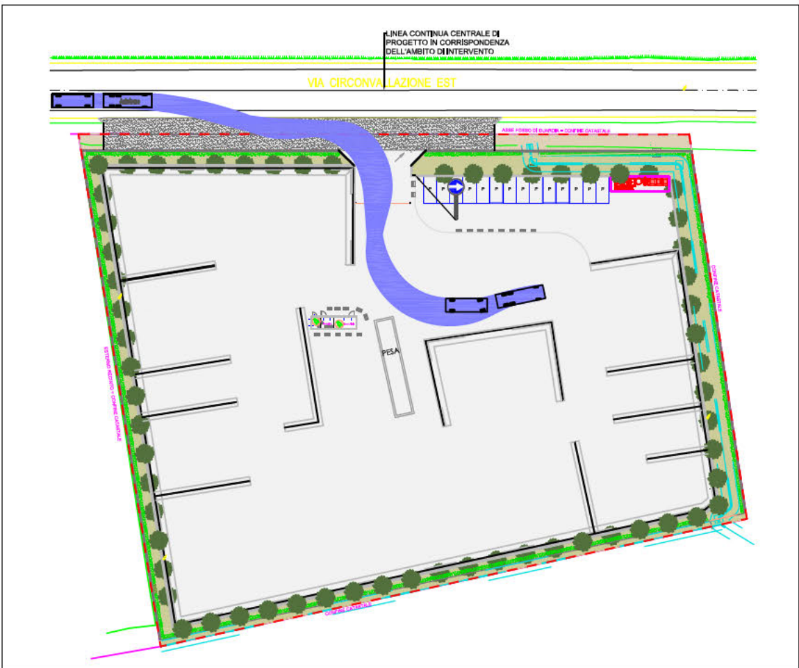
AUTOTRENO MANOVRA IN INGRESSO DA OVEST CON UTILIZZO BANCHINA DI PROGETTO
