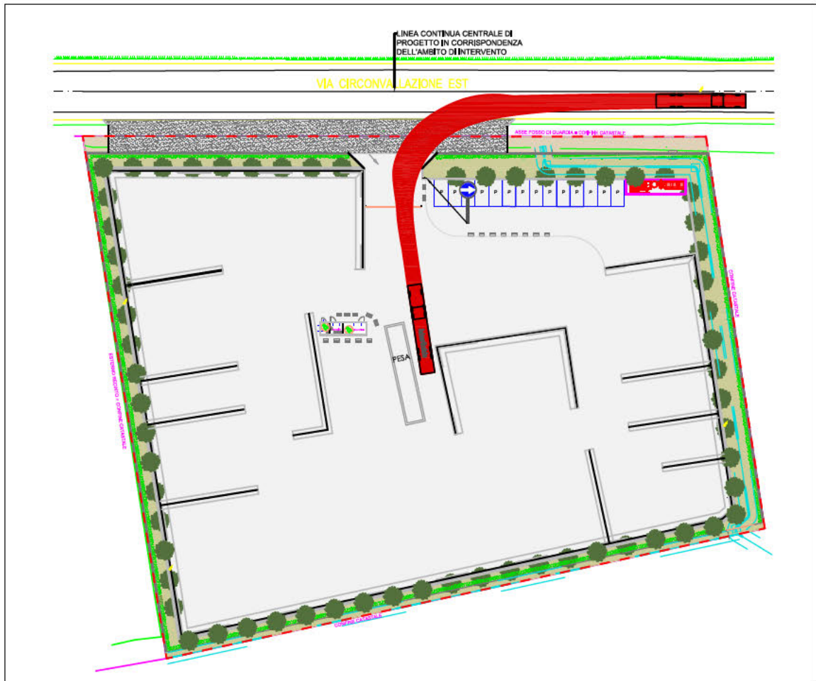
AUTOARTICOLATO MANOVRA IN USCITA VERSO EST
