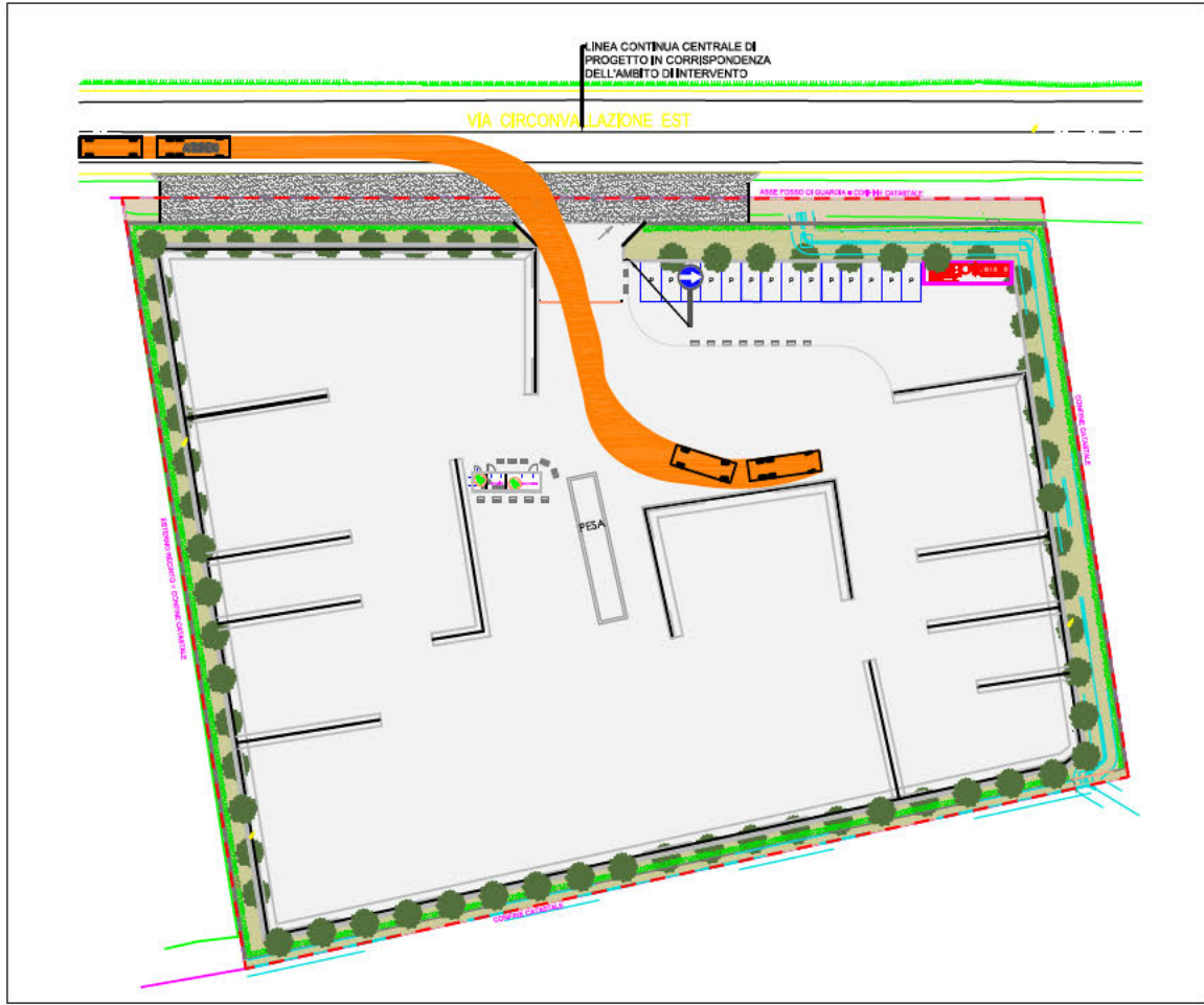
AUTOTRENO MANOVRA IN INGRESSO DA OVEST
