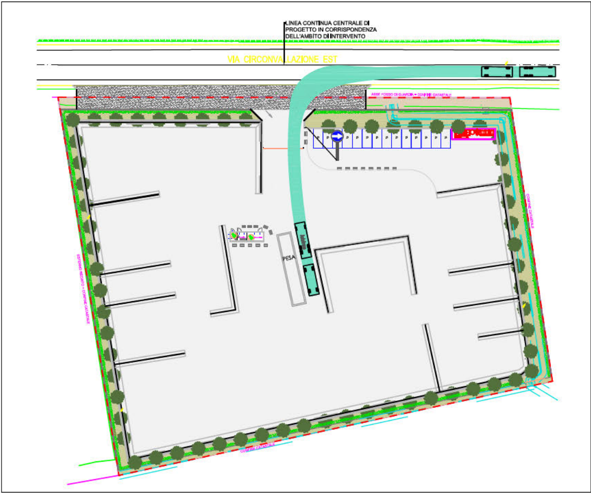
AUTOTRENO MANOVRA IN USCITA VERSO EST
