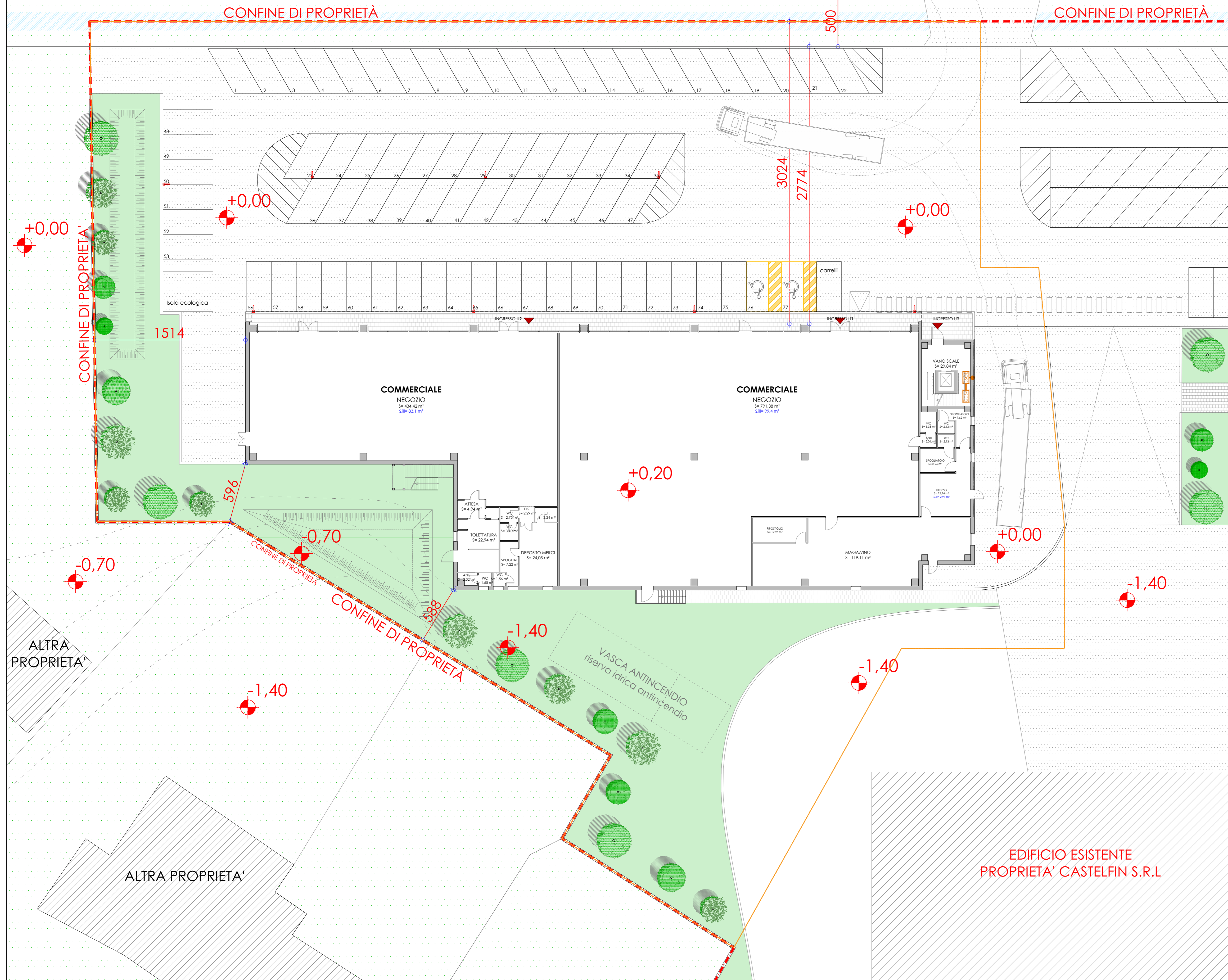
PLANIMETRIA DI PROGETTO scala 1:200
