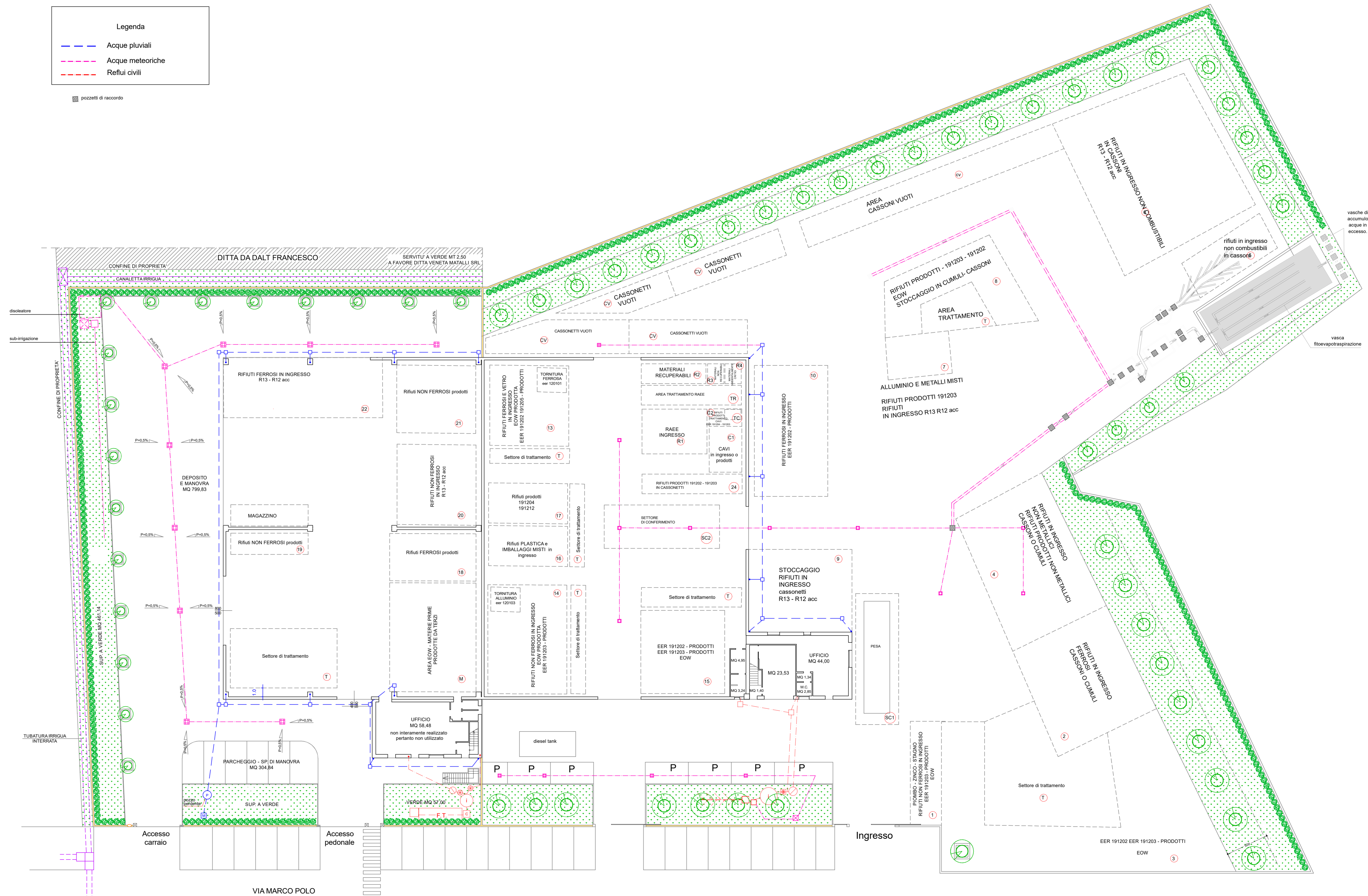
PLANIMETRIA SCALA 1:200
